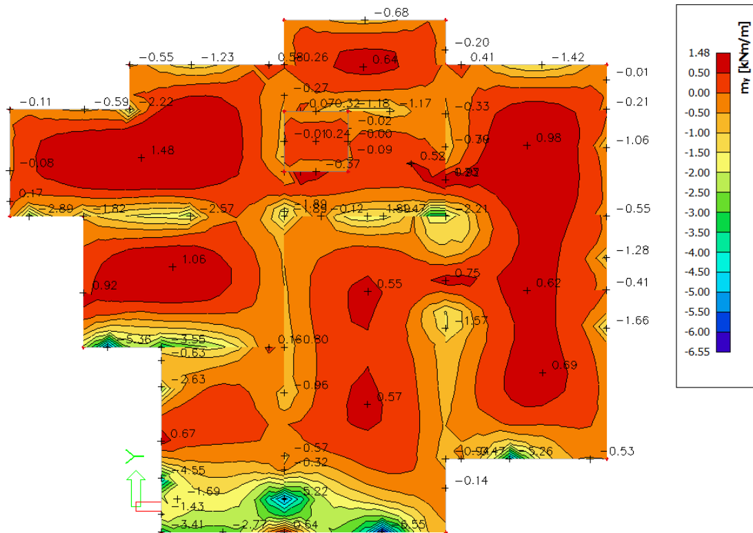
Slika 5.1.6. Prikaz potrebne armature ( cm^2/m ) u smjeru y za GSN1
