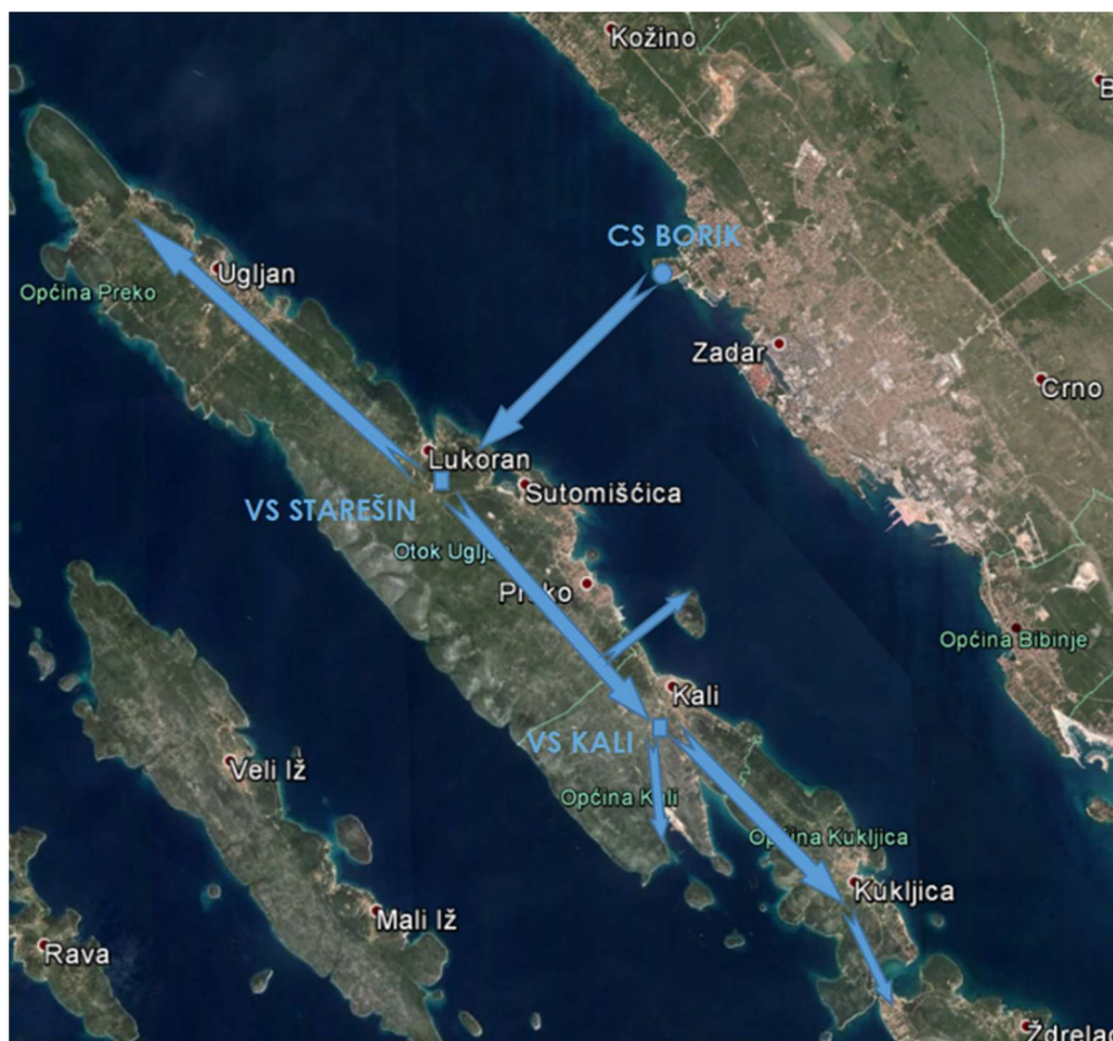
Slika 3: Vodoopskrbni sustav otoka Ugljana
