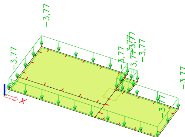
Slika 7.2. Dodatno stalno opterećenje \Delta g=3,77 (kN/m 2 )
