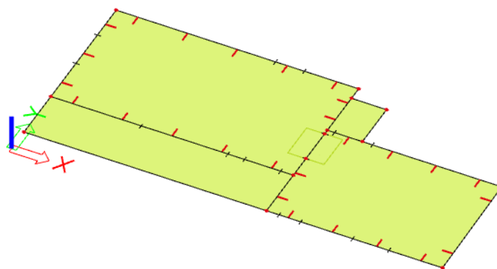
Slika 7.1 Grafički prikaz modela krovne ploče
