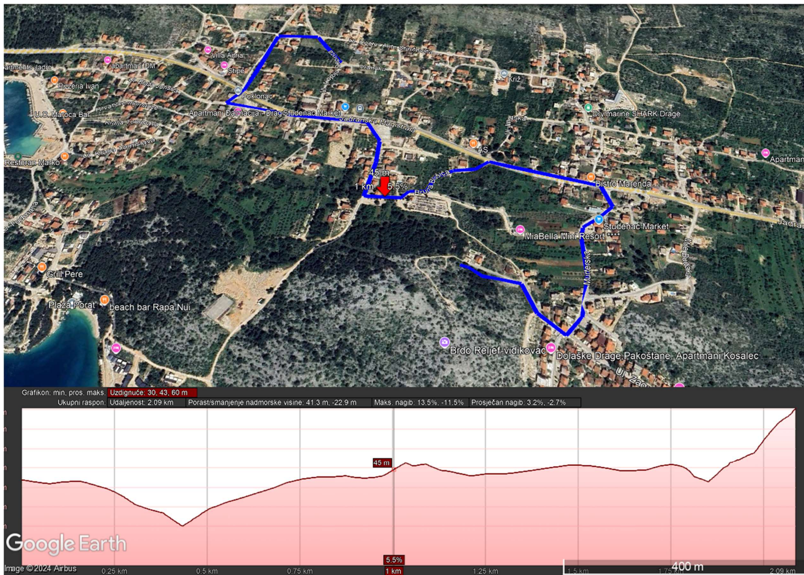
Slika 12. Trasa cjevovoda od precrpne stanice Drage do najnepovoljnijeg čvora 408.
