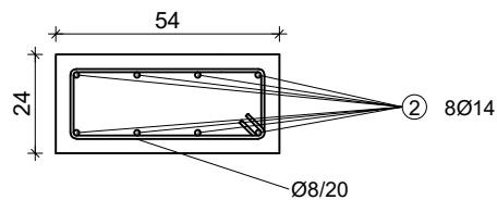
DETALJ ⑤
