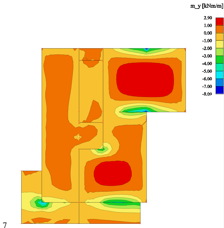
Slika 7.20 Potrebna površina armature A_s(\text{cm}^2/\text{m}) u y smjeru
