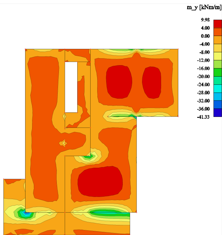
Slika 7.12 Moment savijanja M_{Ed,y} (kNm/m) za GSU-1
