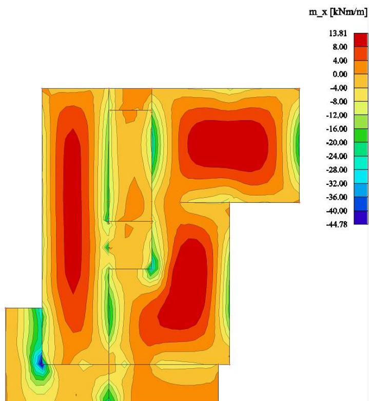
Slika 7.14 Moment savijanja M_{Ed,x} ( \text{kNm/m} ) za GSN-1
