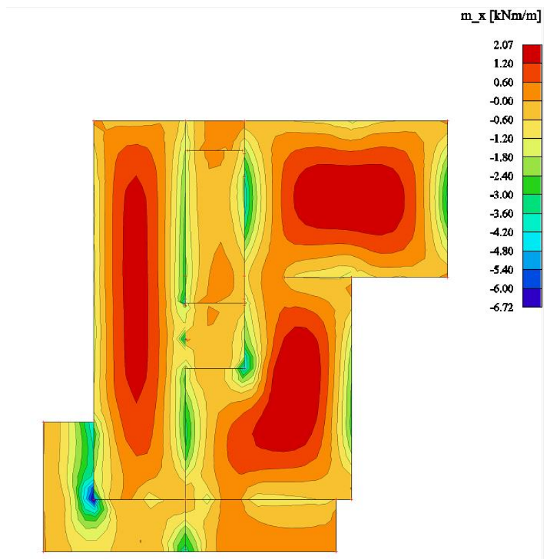
Slika 7.19 Potrebna površina armature A_s(\text{cm}^2/\text{m}) u x smjeru
