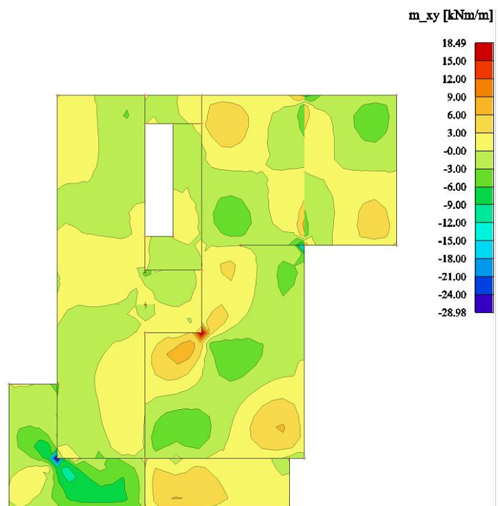
Slika 7.4 Moment savijanja M_{Ed,xy} ( \text{kNm/m} ) za GSN-1
