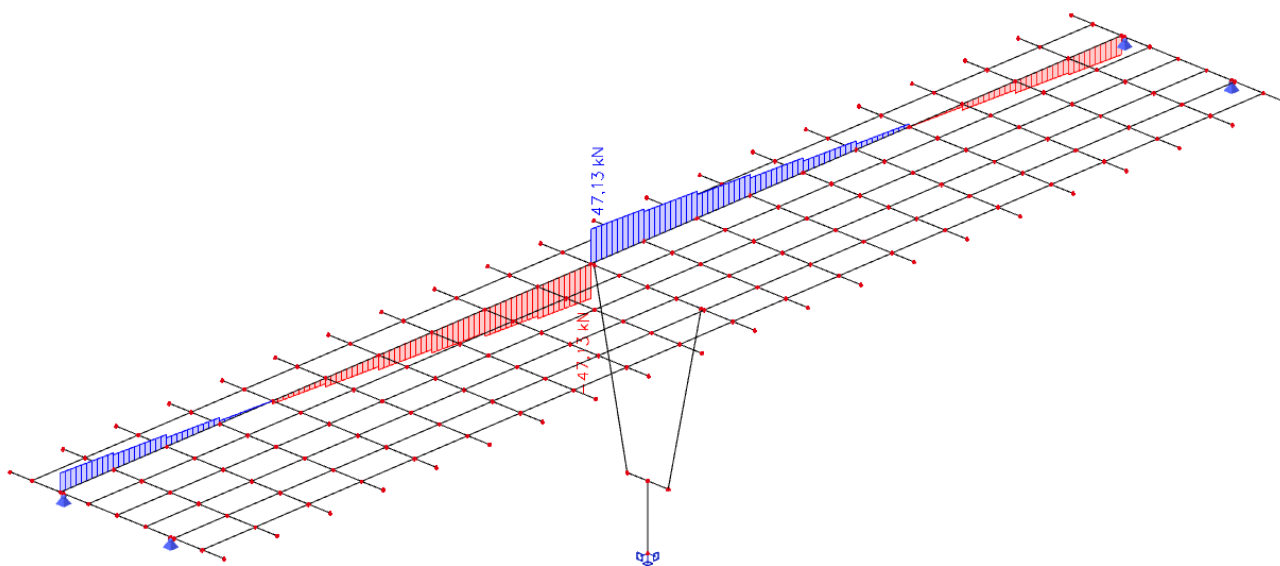
Slika 12: Dodatno stalno opterećenje – poprečna sila ( V_z ) u \text{kN}
