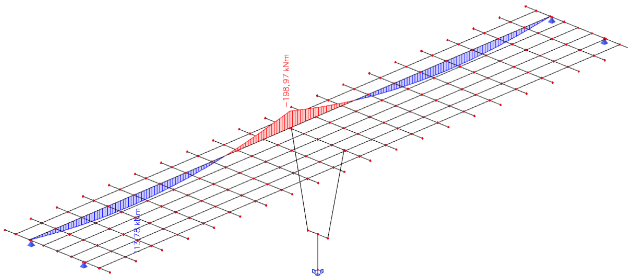
Slika 12: Dodatno stalno opterećenje – momenti savijanja ( M_y ) u \text{kNm}
