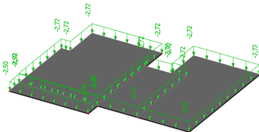
Slika 4.2.1 Dodatno stalno djelovanje G1 [kN/m 2 ]
