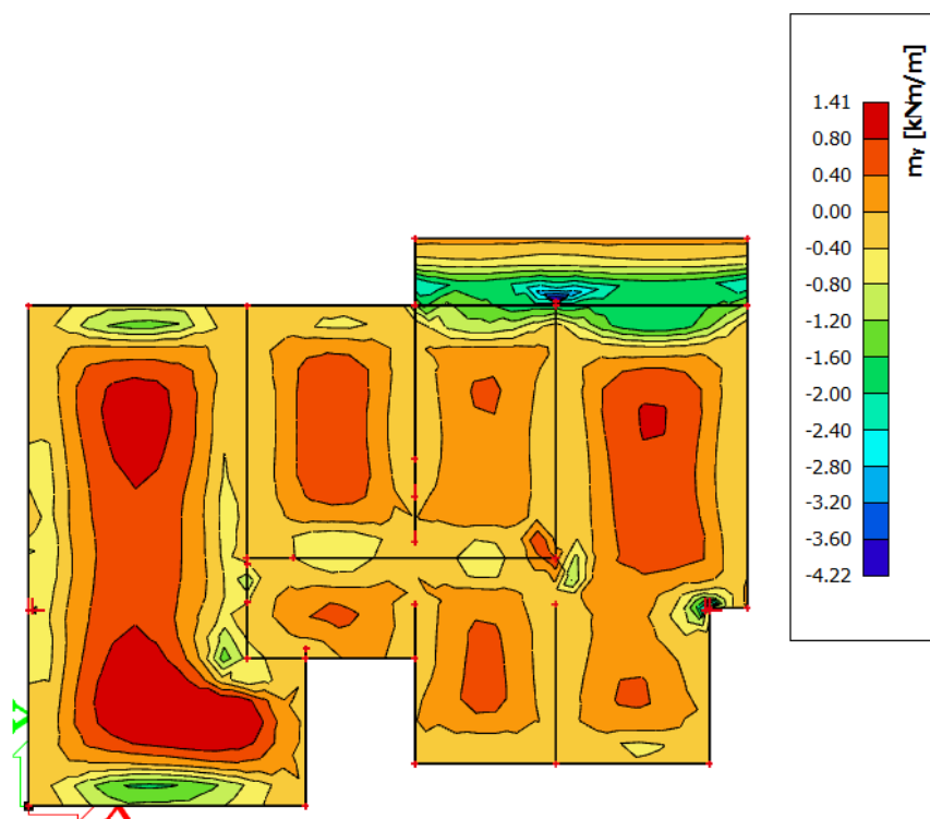
Slika 6.8 Potrebna površina armature A_s (cm 2 /m) u y smjeru
