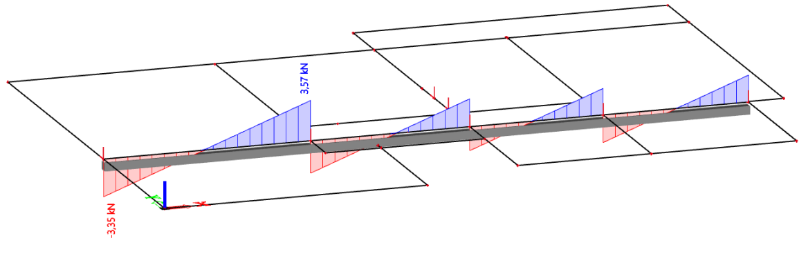
Slika 7.2 Poprečne sile V_{Ed,z} (kN/m) za GSN
