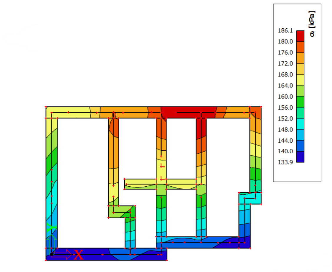
Slika 10.5 Linijske reakcije na mjestima oslanjanja zidova na temeljne trake (Kn/m) za kombinaciju GSN
