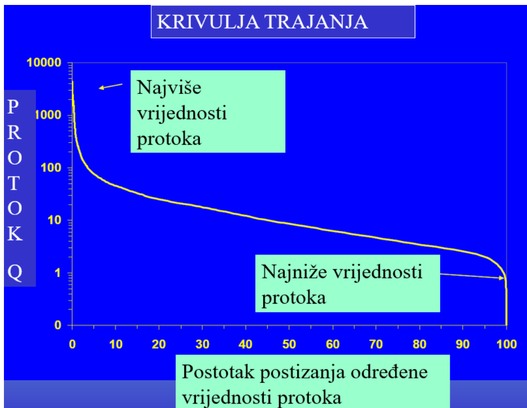
Slika 10: Krivulja trajanja [1]
