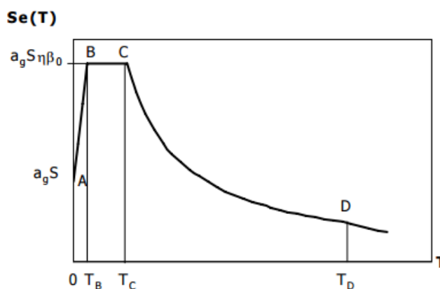
Crtež 4.11. Osnovni oblik elastičnog spektra odgovora za horizontalno seizmičko djelovanje preuzeto iz HRN EN 1998
