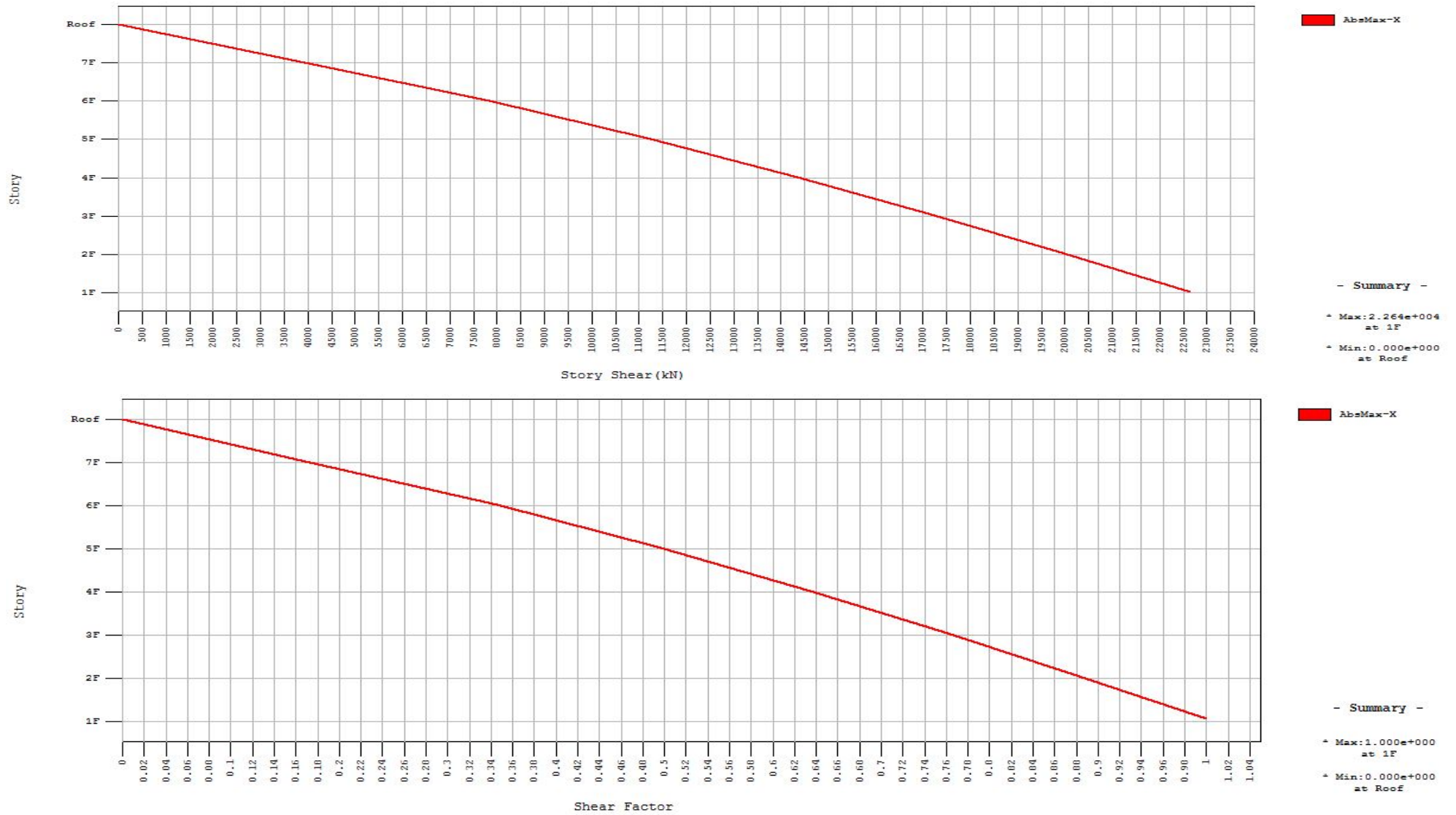
Crtež 5.72. Prikaz raspodjele posmičnih sila po etažama
