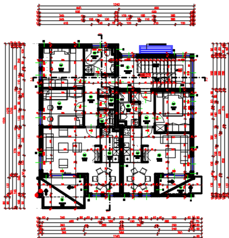
Slika 1.10 Tlocrt 2. kata
