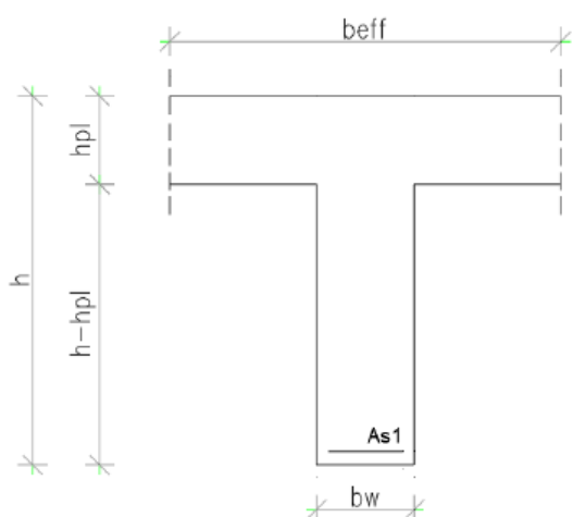
Slika 9.57. Poprečni presjek grede
