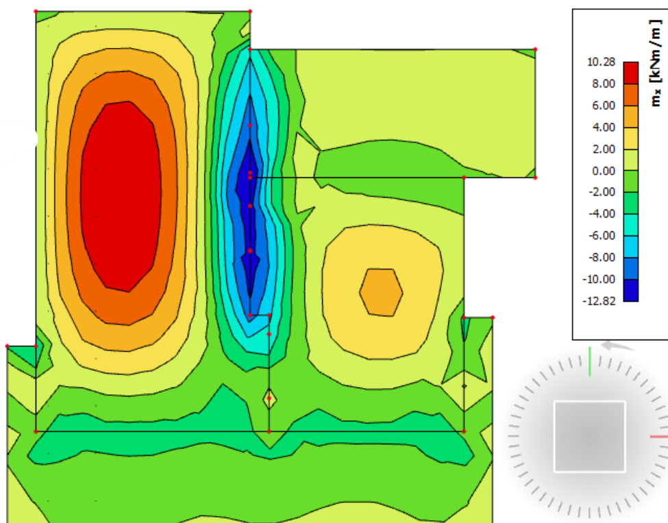
Slika 9.42. Momenti savijanja M_{Ed,x} ( \text{kNm/m} ) za GSU
