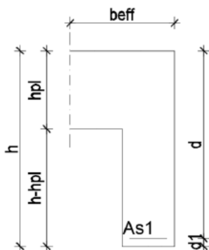
Slika 9.52. Poprečni presjek grede
