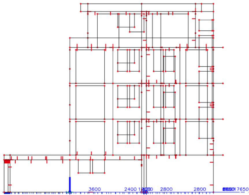
Slika 8.3. Model za proračun (pogled u x smjeru)
