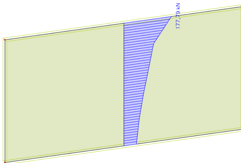
Slika 10.10. Maksimalna poprečna sila za kombinaciju 1,35 \cdot (G + \Delta G) + 1,5Q + 1,35(p_a + p_o)
