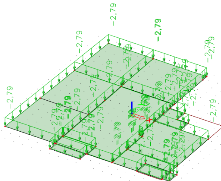
Slika 9.2. Dodatno stalno djelovanje \Delta g=2,79 (kN/m 2 )
