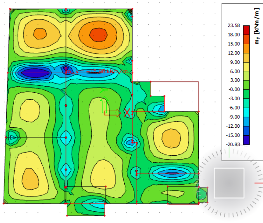
Slika 9.5. Moment savijanja M_{Ed,y} (kNm/m) za GSN-1
