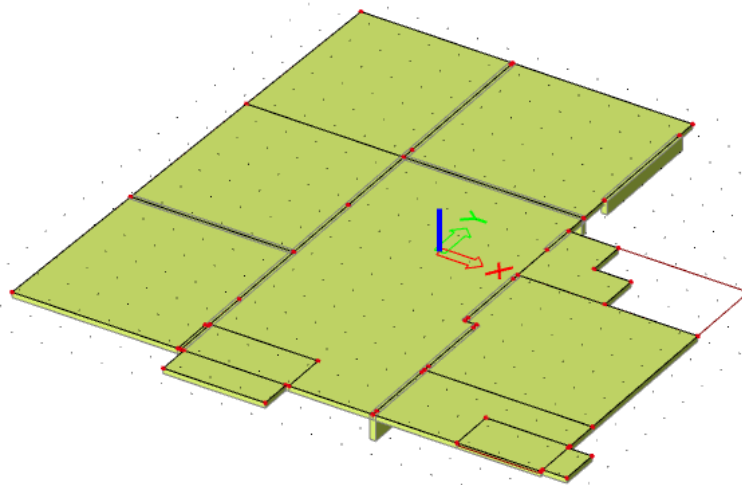
Slika 9.1. Prikaz pozicije 100
