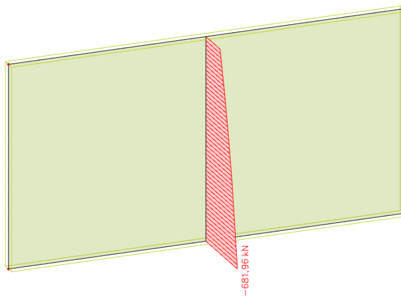
Slika 10.9. Maksimalna uzdužna sila za kombinaciju 1,35 \cdot (G + \Delta G) + 1,5Q + 1,35(p_a + p_o)
