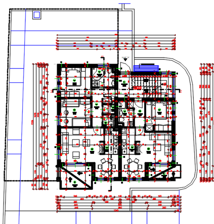
Slika 1.8 Tlocrt prizemlja
