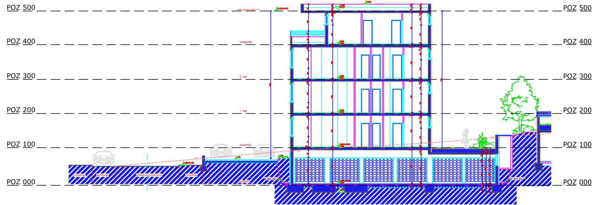
PRESJEK 1-1
