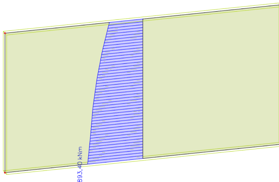
Slika 10.8. Maksimalni moment za kombinaciju 1,35 \cdot (G + \Delta G) + 1,5Q + 1,35(p_a + p_o)
