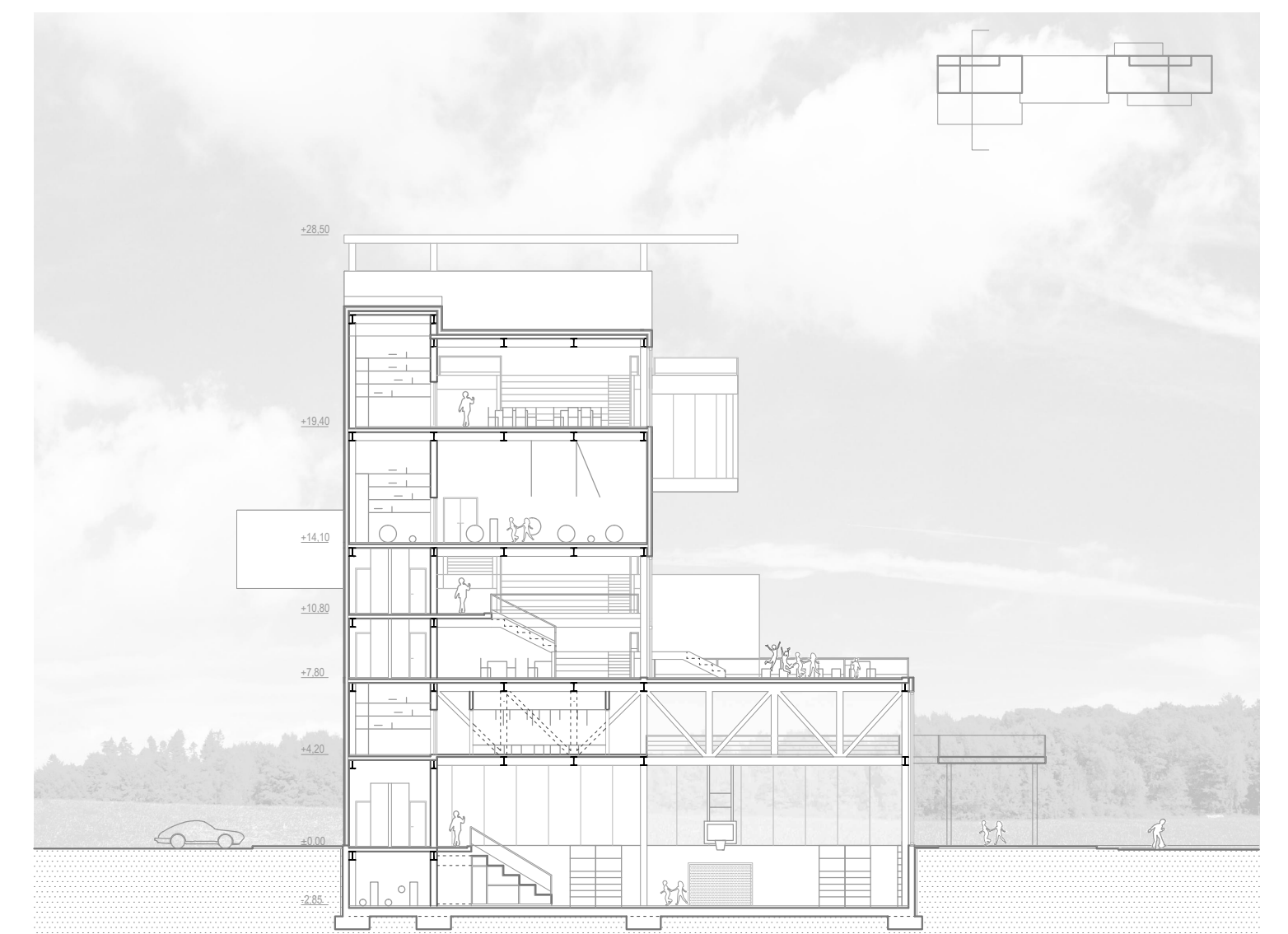
PRESJEK
