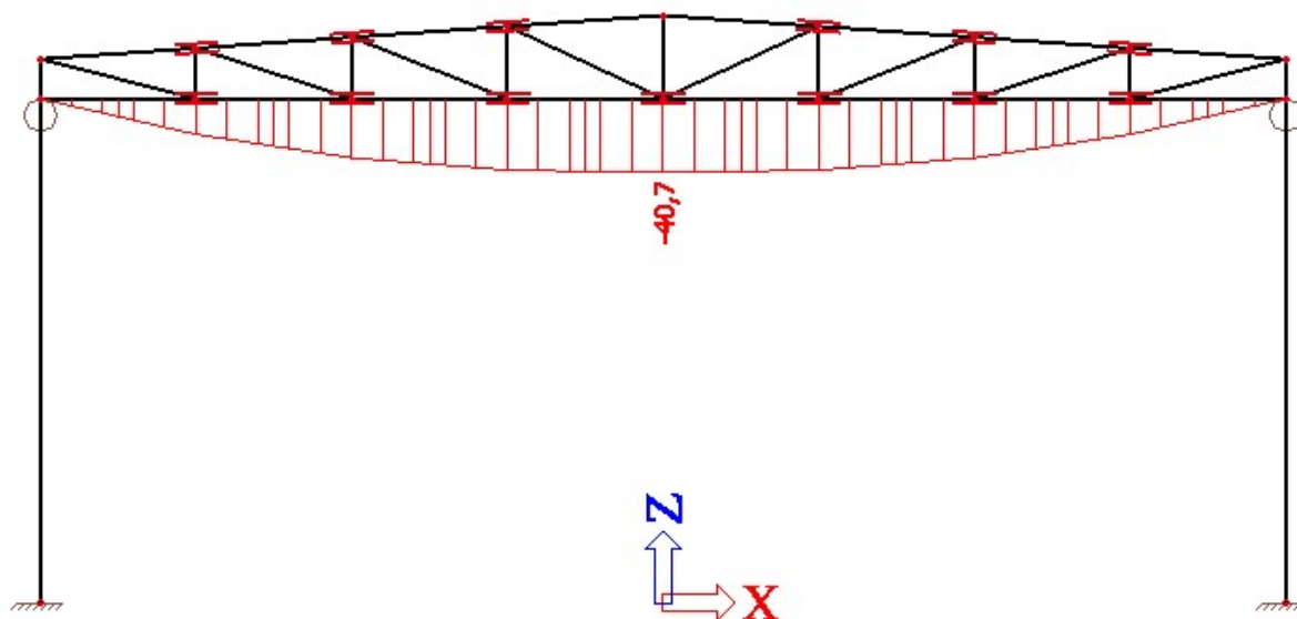
Slika 9. Vertikalni progib rešetke
