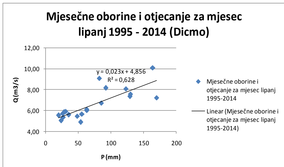
Slika 9.21. Regresija između mjesečnih oborina i srednjih mjesečnih protoka za mjesec lipanj
