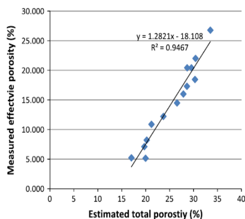
Slika 3.7. Veza između efektivne i ukupne poroznosti[14]
