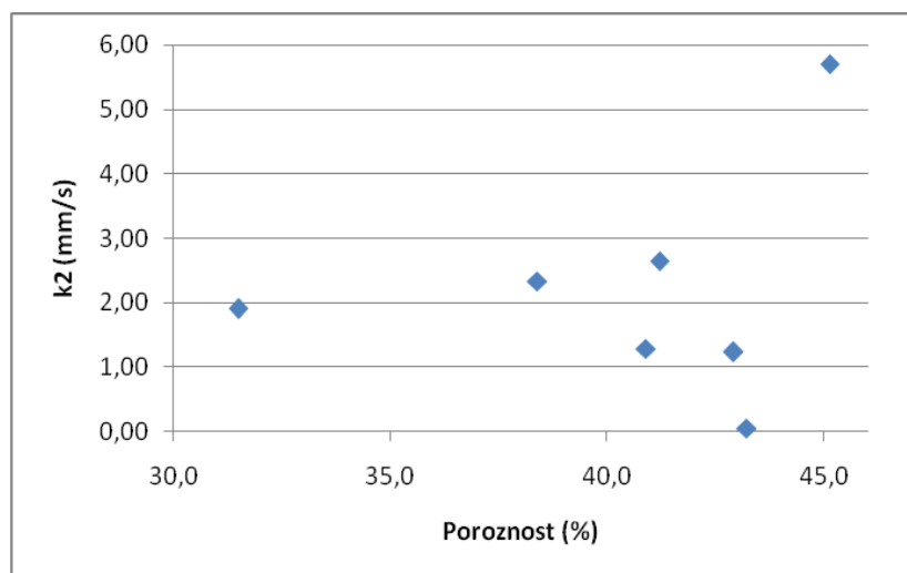
Slika 4.39. Veza između k_2 i poroznosti
