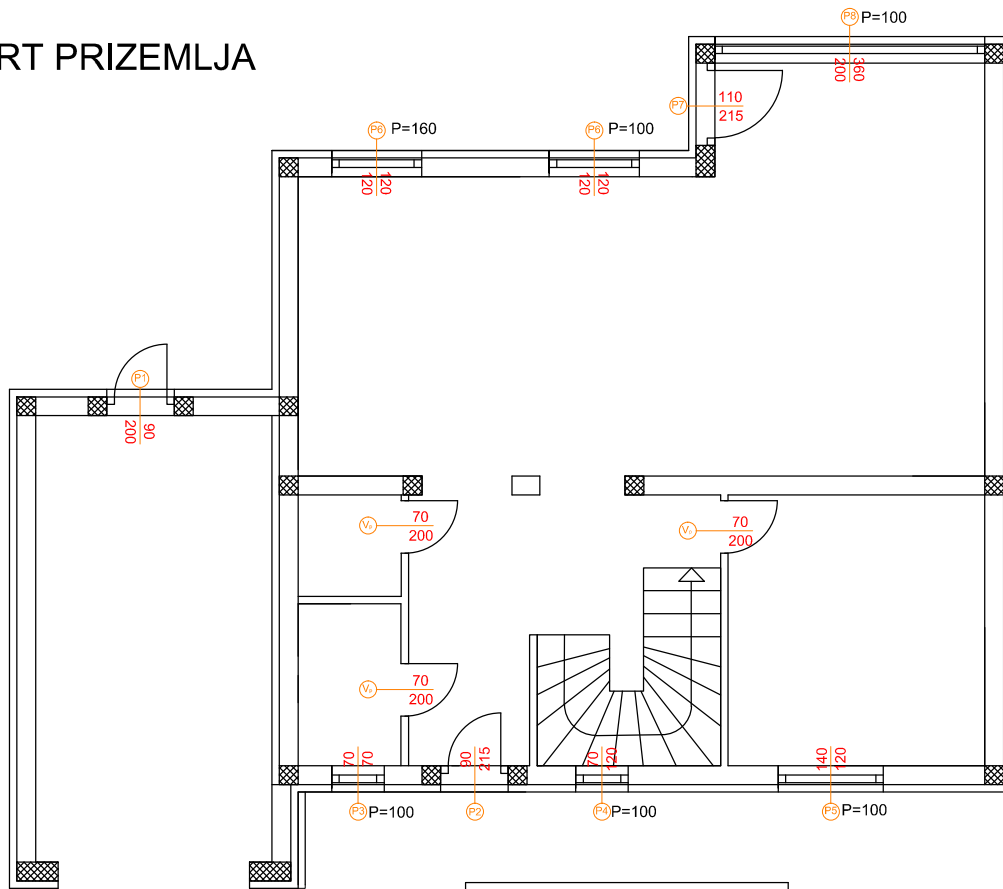
TLOCRT KATA
