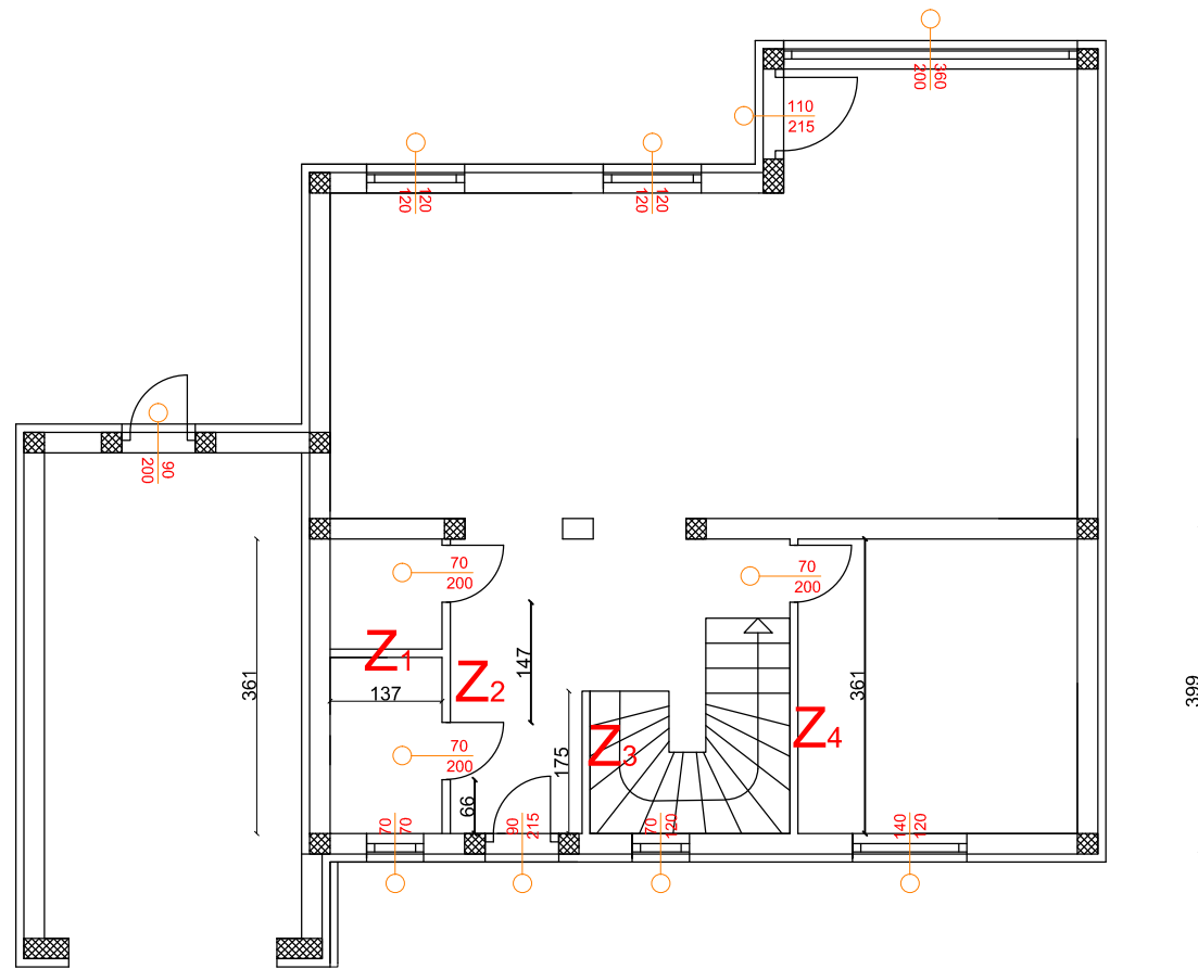
TLOCRT PRIZEMLJA
