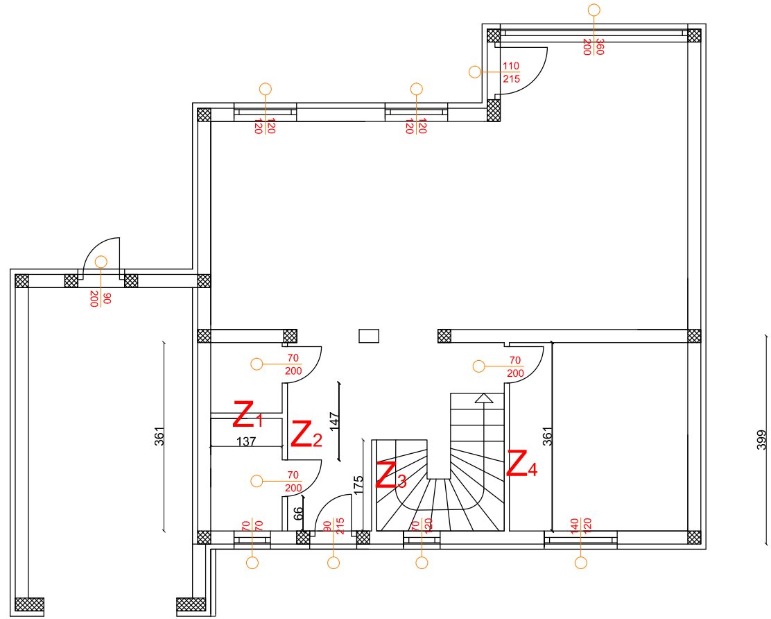
TLOCRT PRIZEMLJA
