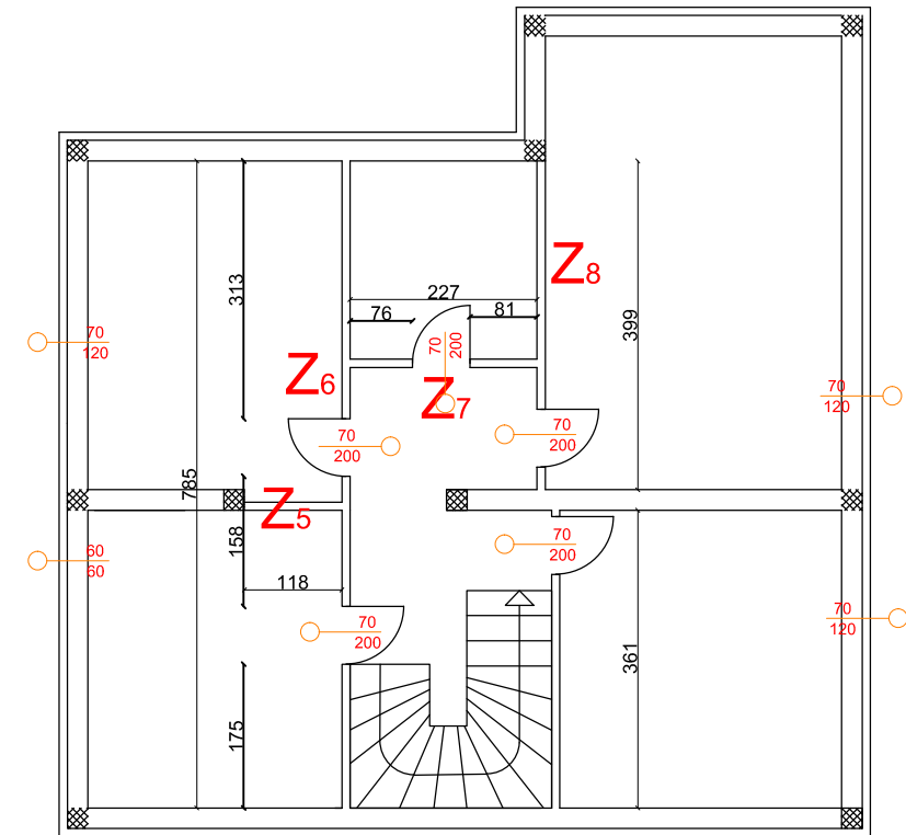
TLOCRT KATA
