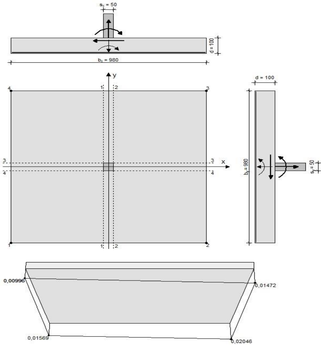
Slika 6.17. Dimenzije temelja i prikaz naprezanja
