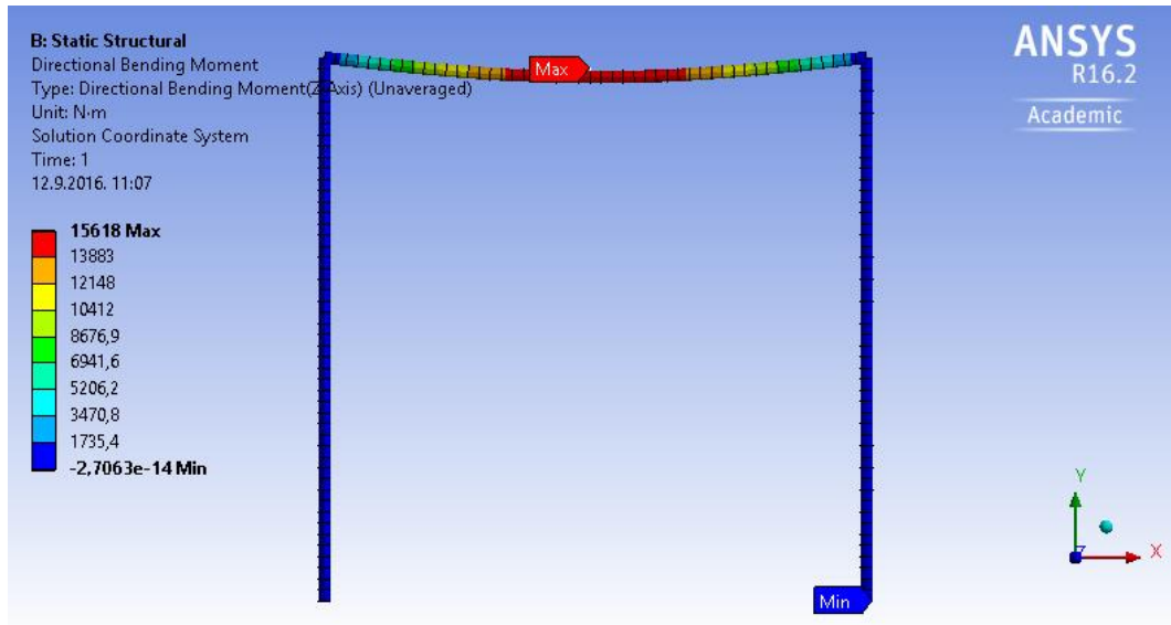
2.2 Momenti savijanja u ravnini okvira [Nm]
