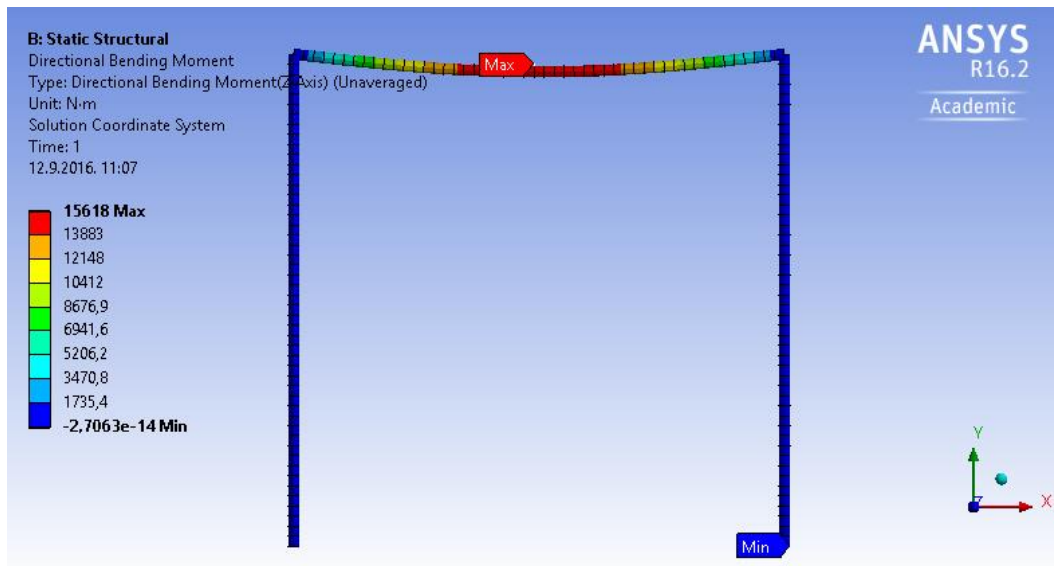
2.2 Momenti savijanja u ravni okvira [Nm]
