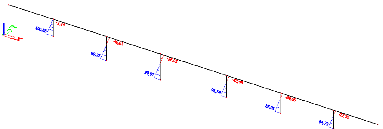
Slika 1.58. - Poprečna sila V_z (vjetar uzdužno na prazni most)
