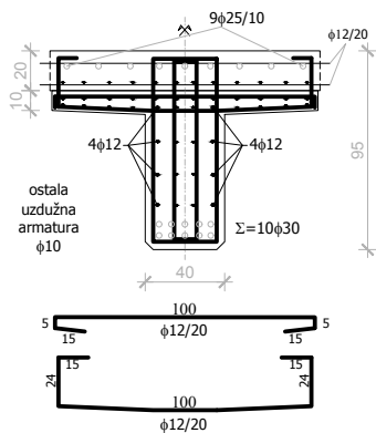
Poprečni Presjek nosača
