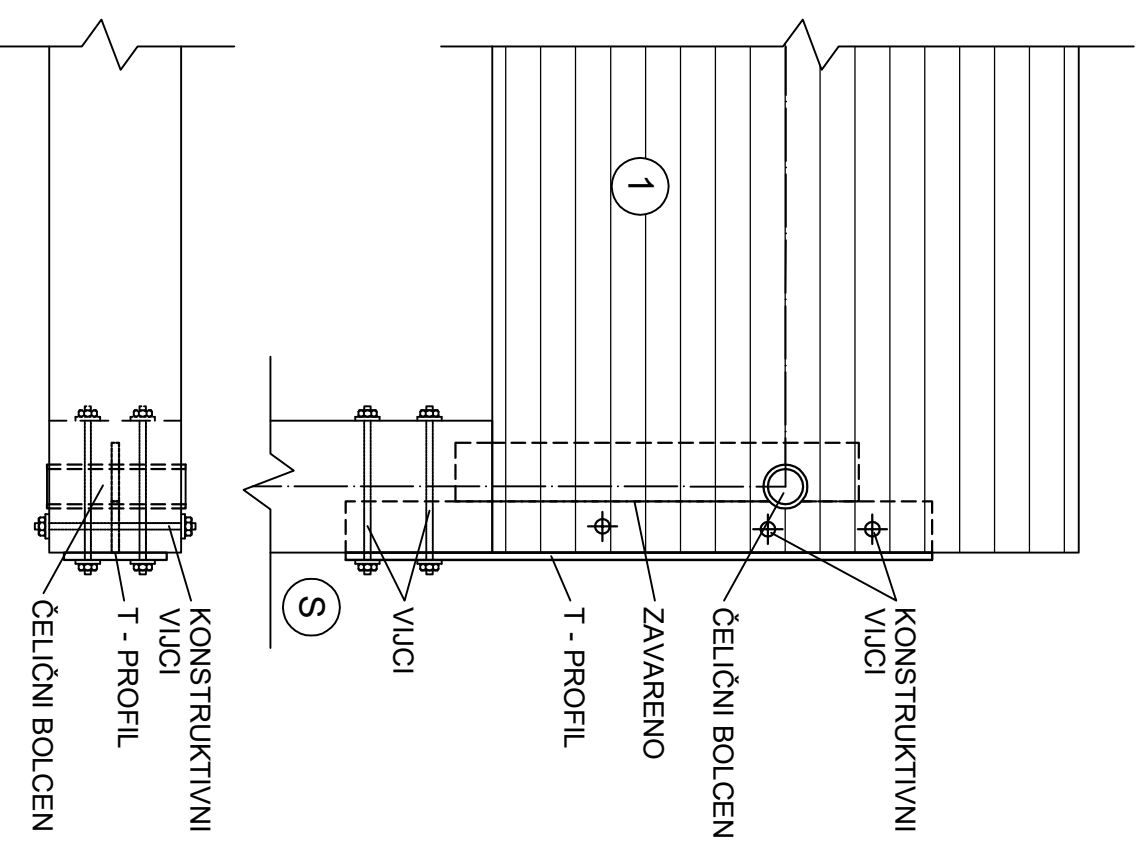
SPOJ STUP - LAMELIRANI NOSAČ
