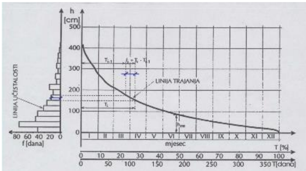
Slika 3.3.1. Prikaz krivulje trajanja i krivulje učestalost - Izvor [6]
