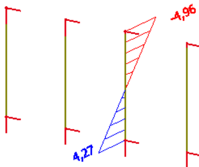
Slika 5.2. Maximalni moment savijanja M za kombinaciju 1,35G+1,5Q+1,5\cdot 0,6W_y za stupove 20/25 u prizemlju
