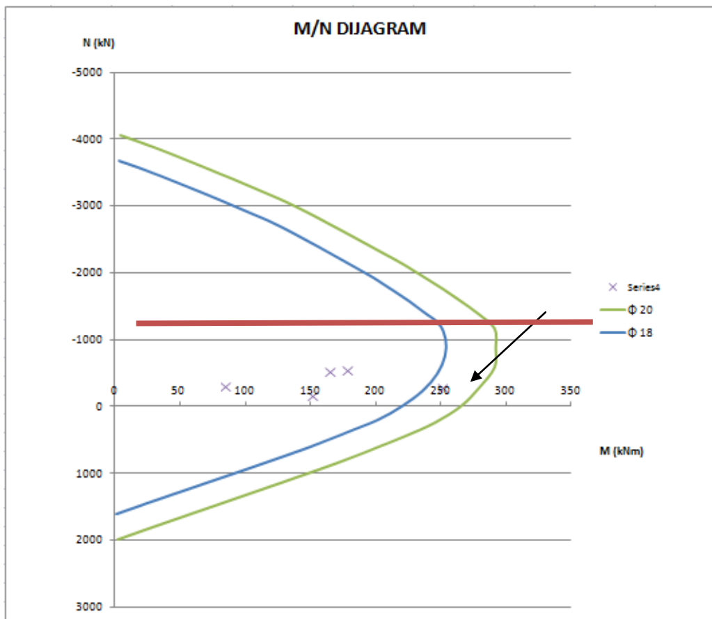
Slika 199: Dijagram stupa SP 1
