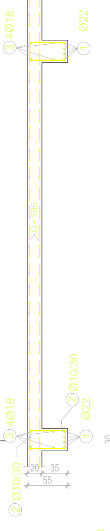
Detalj 1 M 1:50
