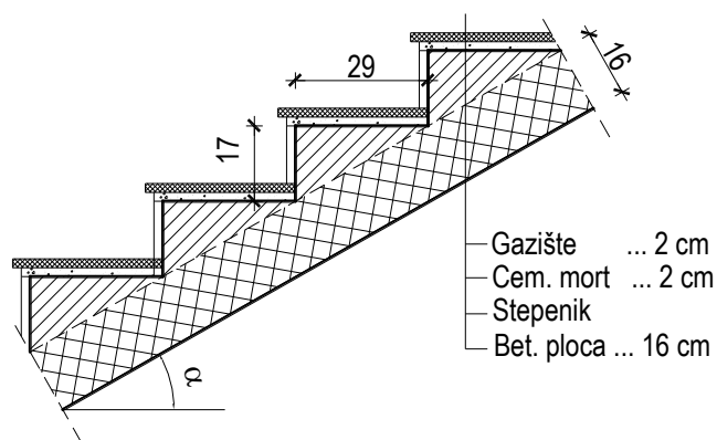
Slika 1: Geometrija stubišta
