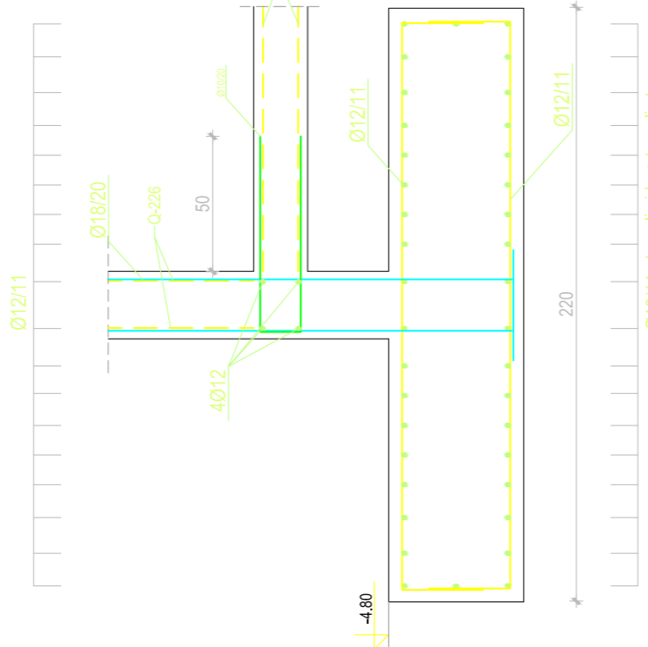
PRESJEK 2 - 2
