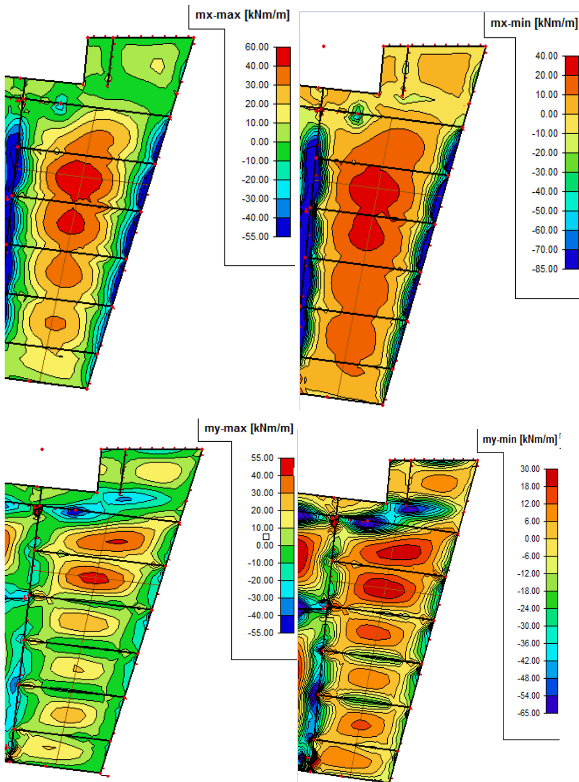
Slika 36: Prikaz maksimalnih i minimalnih momenata savijanja pozicije 103
