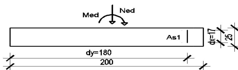
Slika 67: Skica poprečnog presjeka zida
