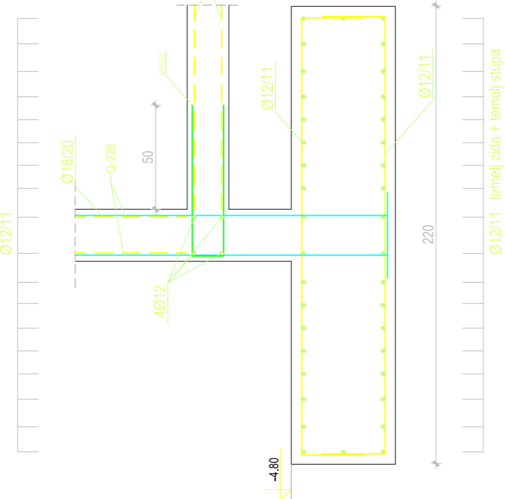
PRESJEK 2 - 2
