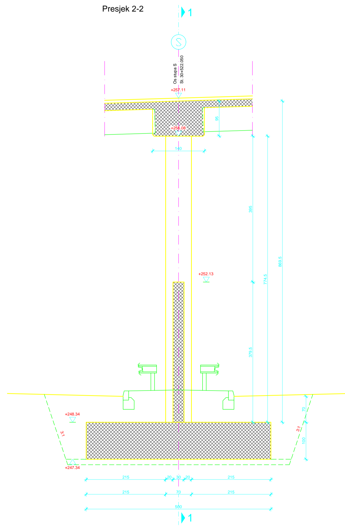
Presjek 2-2
