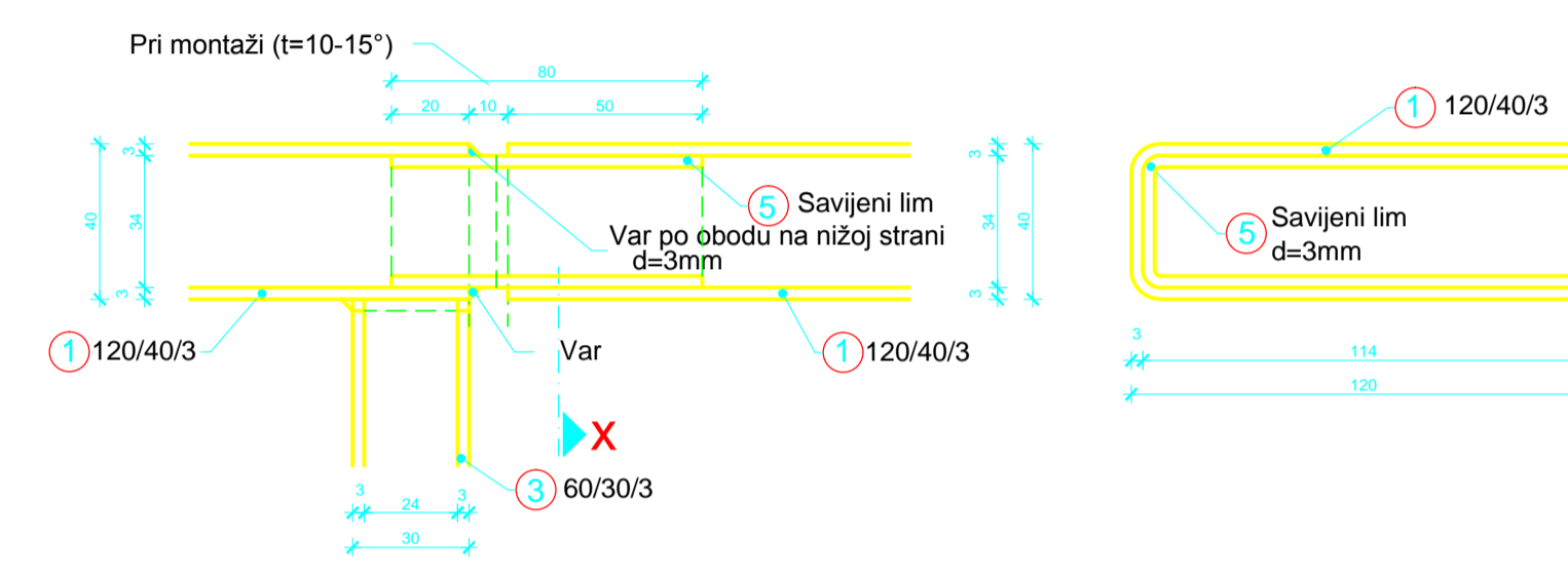
Detalj D1 1:2
