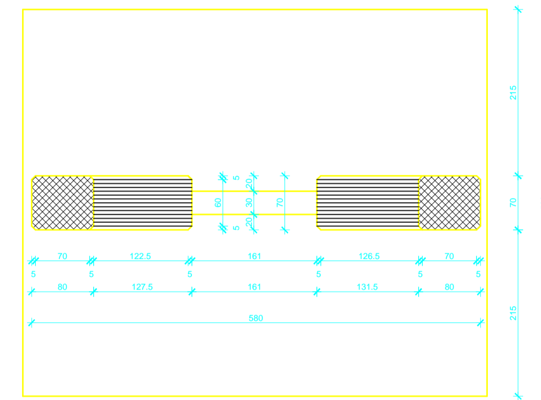
Presjek 4-4
