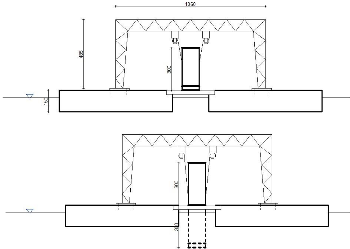
Slika 38. Shematski prikaz betoniranja stupova
