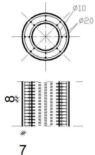
Slika 39. Armatura stupa
