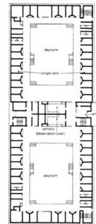
Slika 9: PDBS zatvor (1992), predloženi presjek i tlocrt
