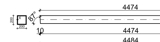
POZ 5b 200x200x7.1, L= 4484 mm, kom 1
