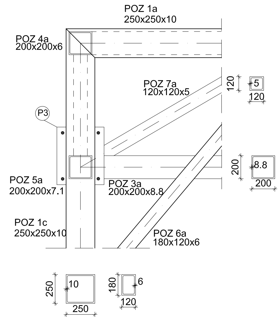
PRESJEK 2-2
