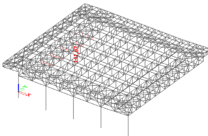
Crtež 8.17. Mjerodavna uzdužna sila u zaštićenju podrožnici od požarne kombinacije
