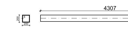
POZ 5e 200x200x7.1, L= 4307 mm, kom 1
