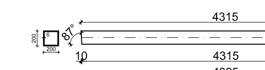
POZ 5d 200x200x7.1, L= 4325 mm, kom 1
