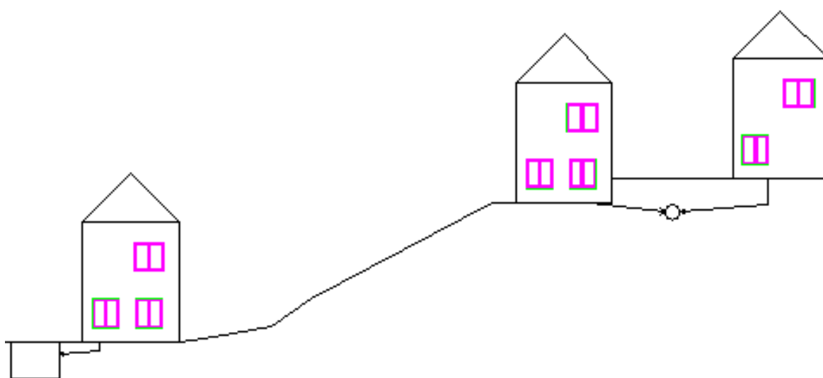
Slika 15.4.2. Karakteristični presjek Dubrovačke ulice
