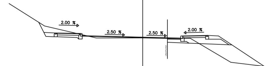
Presjek 3, STACIONAŽA 0+40.00
