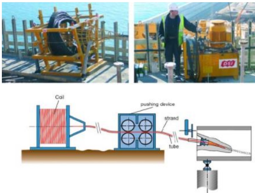
Slika 2.13. Uvlačenje užadi [11]
