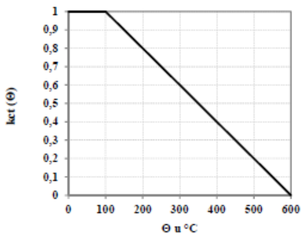
Slika 3.2. Koeficijent k_c(\theta) kojim se uzima u obzir umanjnje vlačne čvrstoće betona, f_{ctk} , pri povišenim temperaturama [5]
