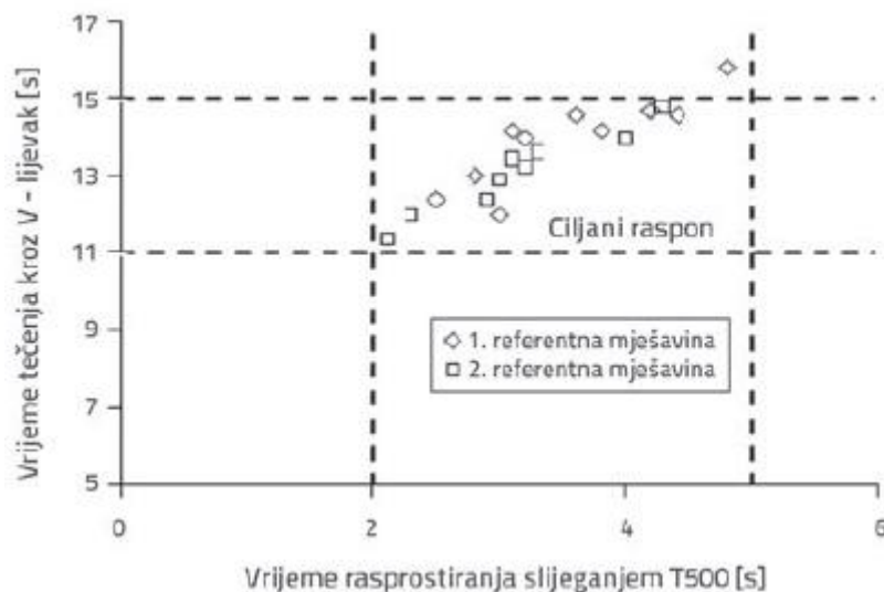
Slika 4.3. Odnos vremena potrebno za rasprostiranje slijevanjem od 500 mm i tečenja kroz V-lijevak [14]
