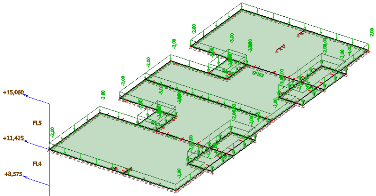
Slika 33: pokretno opterećenje(q)
