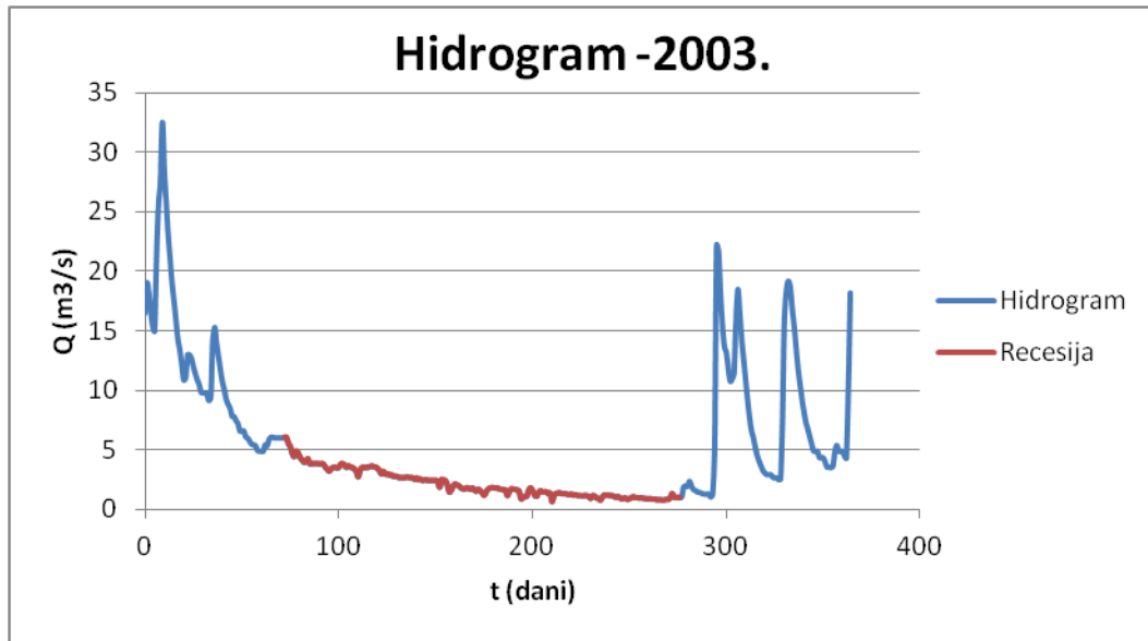
Slika 5.24. Hidrogram i recesija rijeke Vrljike za 2003.g.
