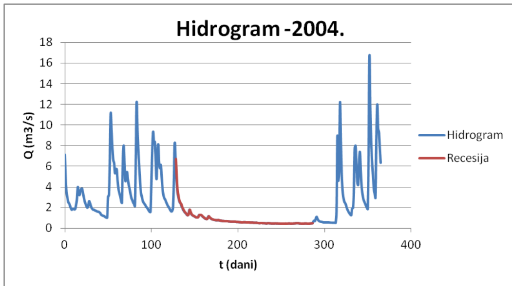
Slika 5.20. Hidrogram i recesija rijeke Žrnovnice za 2004g.
