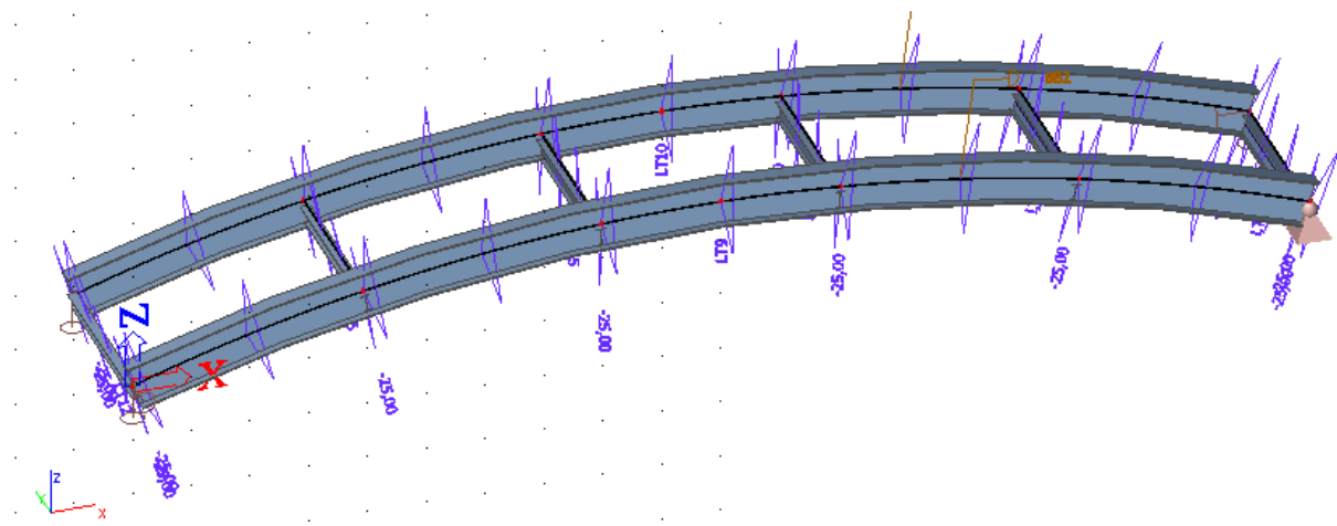
Slika 9.. Raspodjela temeteraturnog opterećenja – skupljanje
