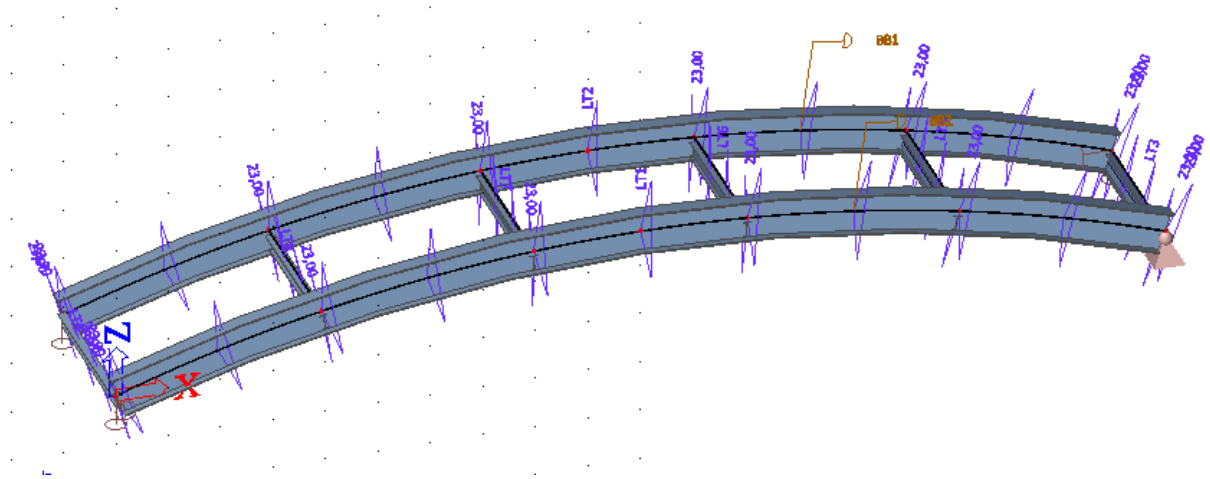
Slika 8.. Raspodjela temeteraturnog opterećenja – širenje
