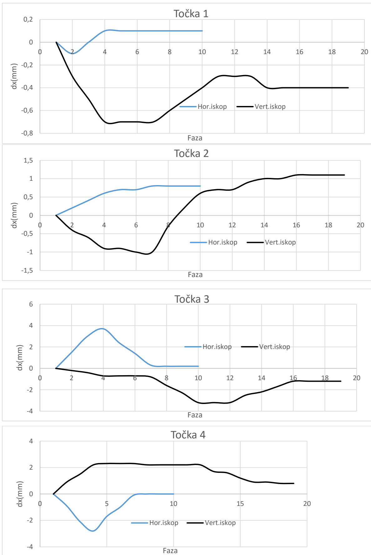
Slika 87. Usporedba pomaka točkaka 1,2,3,4 dx (mm)
