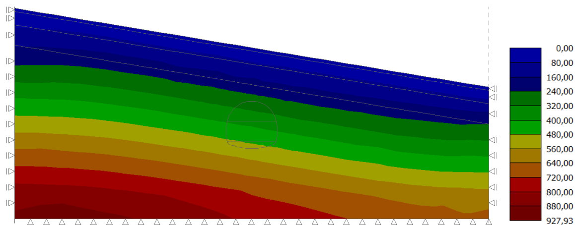
Slika 14. Naprezanja u tlu \sigma_z (kPa)
