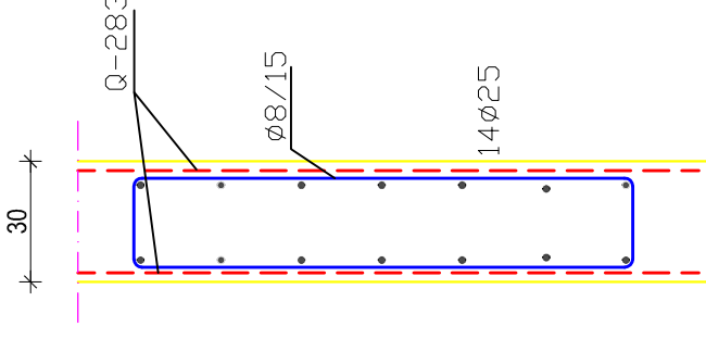
Detalj B
