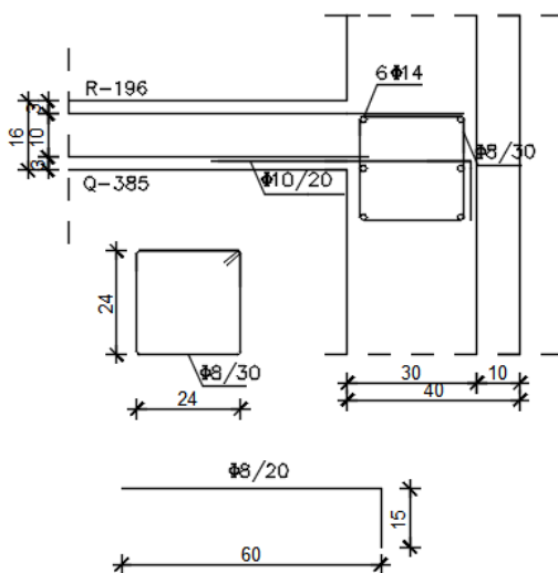
presjek 1-1
