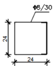
DETALJ 3
