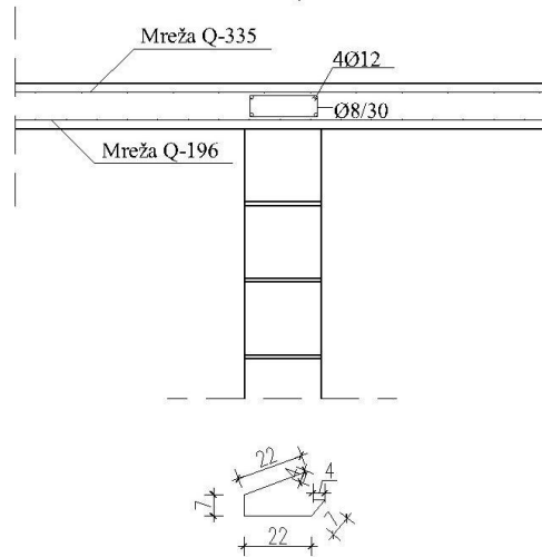
Presjek 2-2
