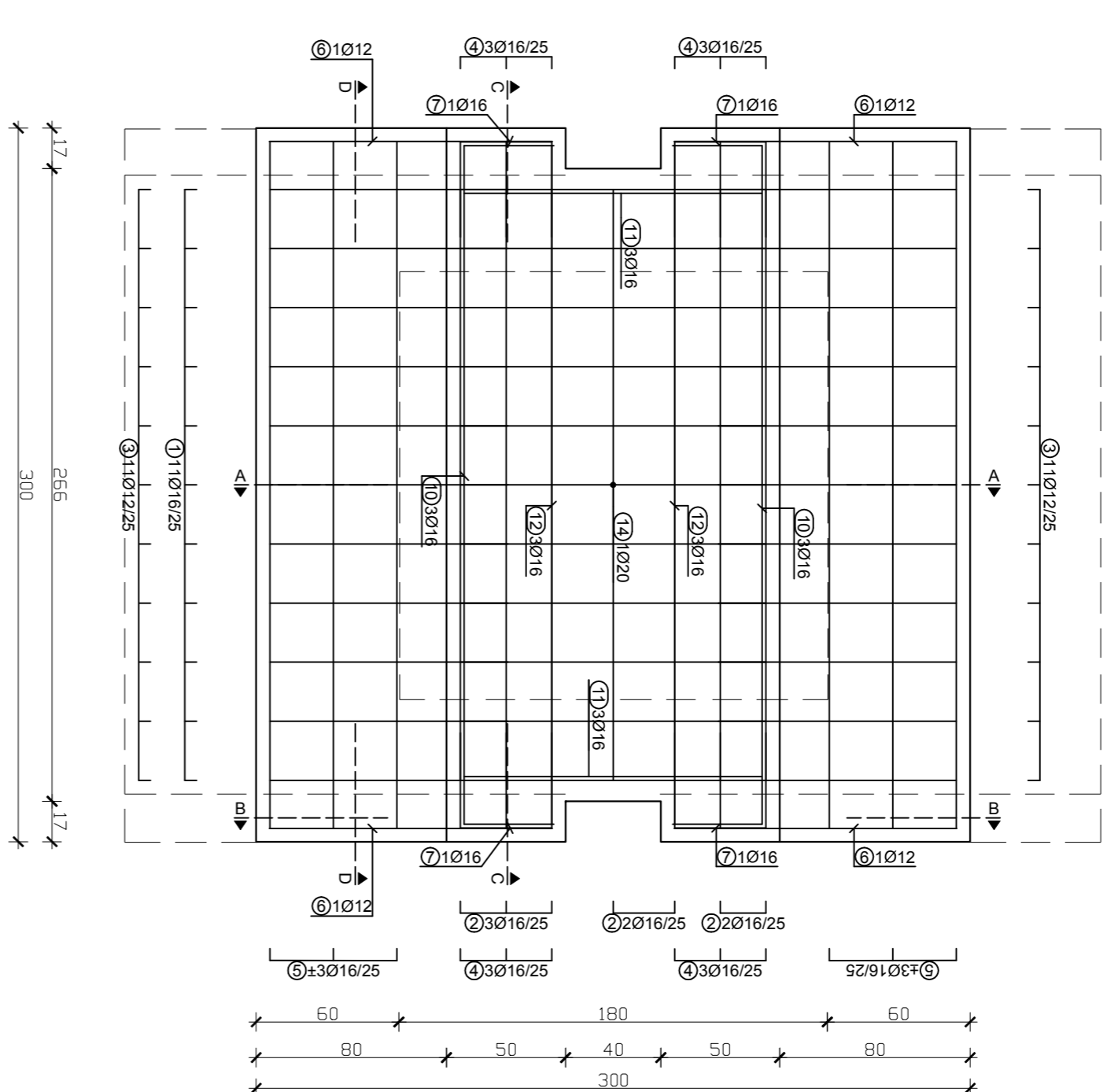
TLOCRT DO KOTE +0,75
