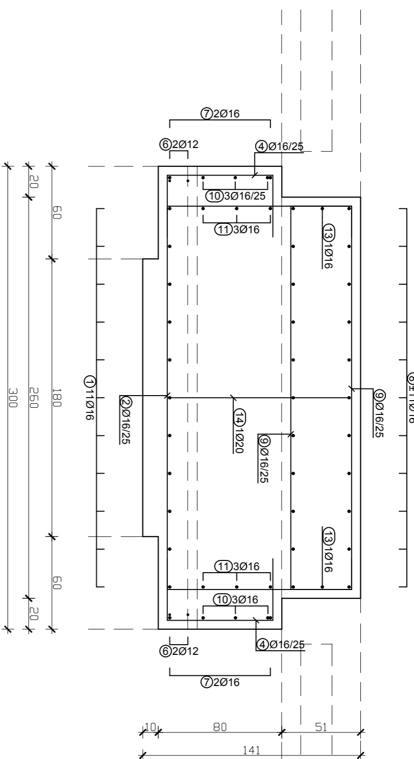
PRESJEK C-C
