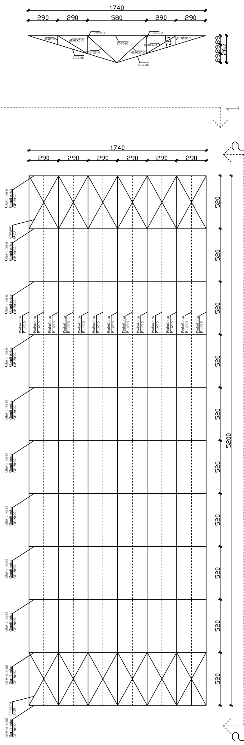
UZDUŽNI POGLED 2-2
