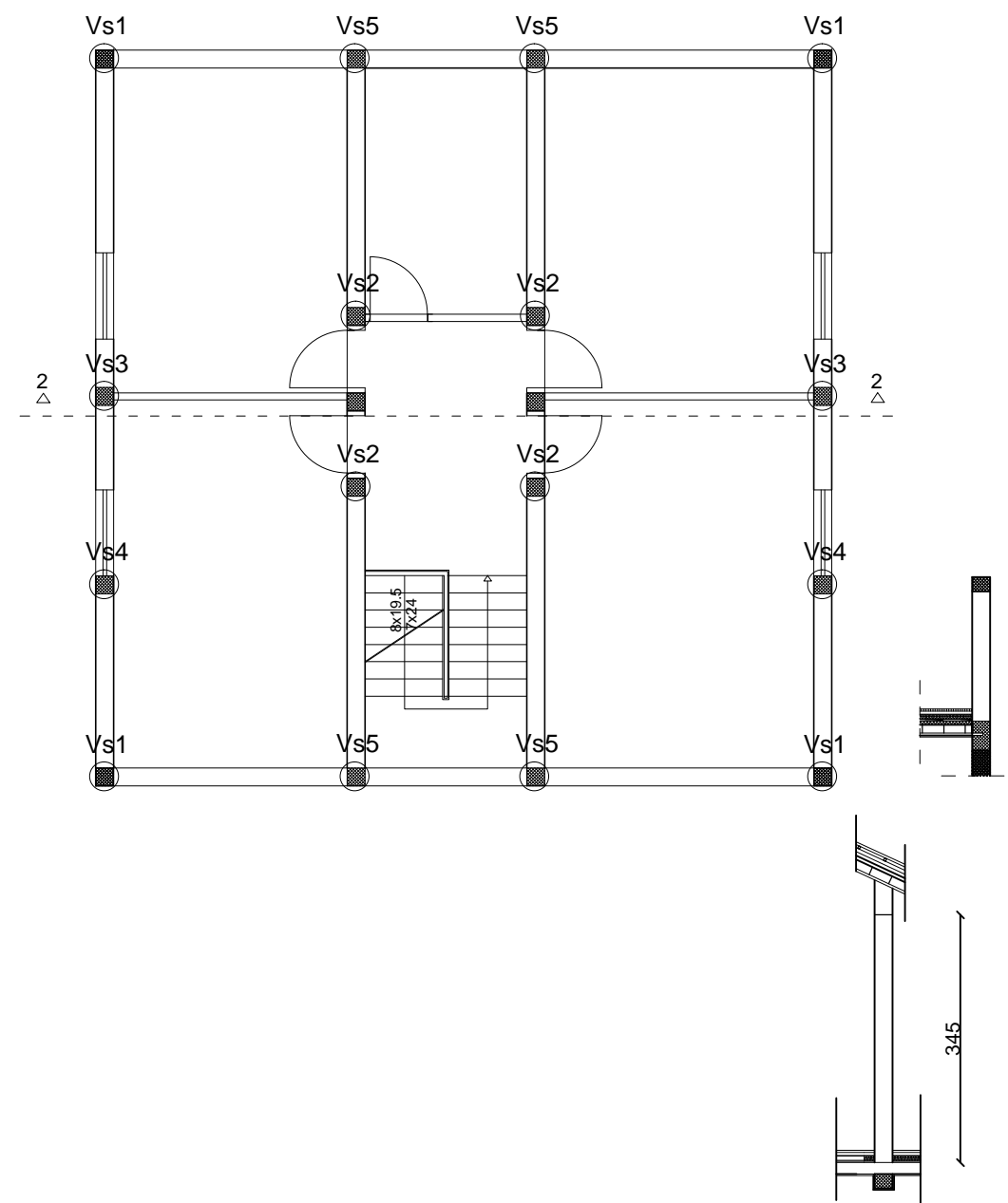
TLOCRT KATA
