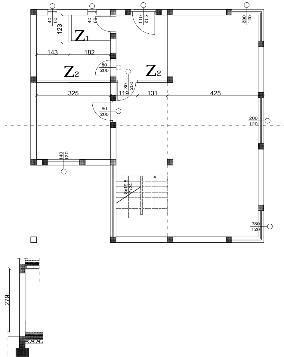
TLOCRT PRIZEMLJA
