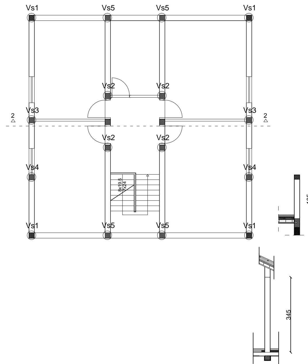
TLOCRT KATA
