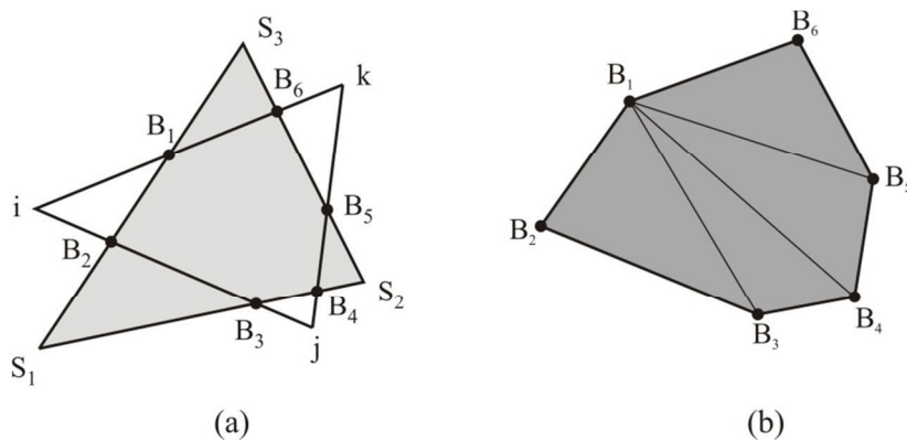
Crtež 3.5 Kontaktni poligon (a) presječnica (b) izračun kontaktnih sila [M12]
