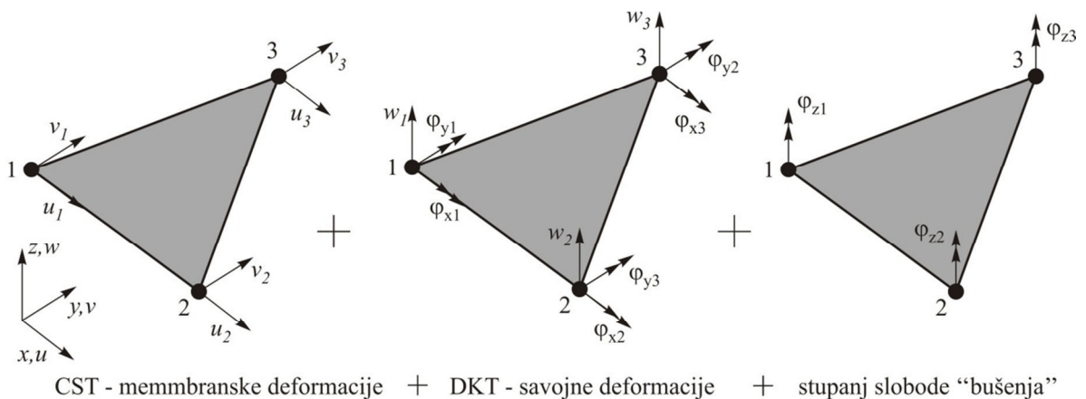
CST - membranske deformacije + DKT - savojne deformacije + stupanj slobode "bušenja"
