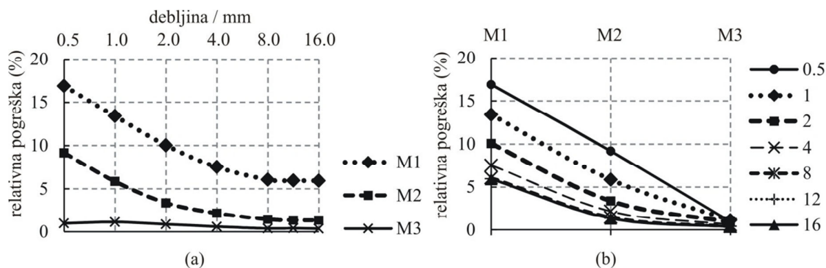
Crtež 5.30 Kružna ploča (a) ovisnost pogreške o debljini za različite diskretizacije (b) ovisnost pogreške o diskretizaciji za različite debljine
