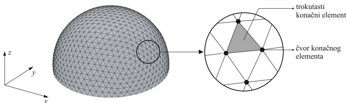
Crtež 5.1 Diskretizacija konstrukcije ljuske
