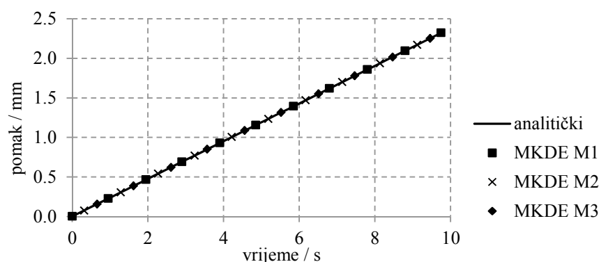
Crtež 5.20 Usporedba analitičkog i numeričkog pomaka na desnom kraju vlačno opterećene ploče
