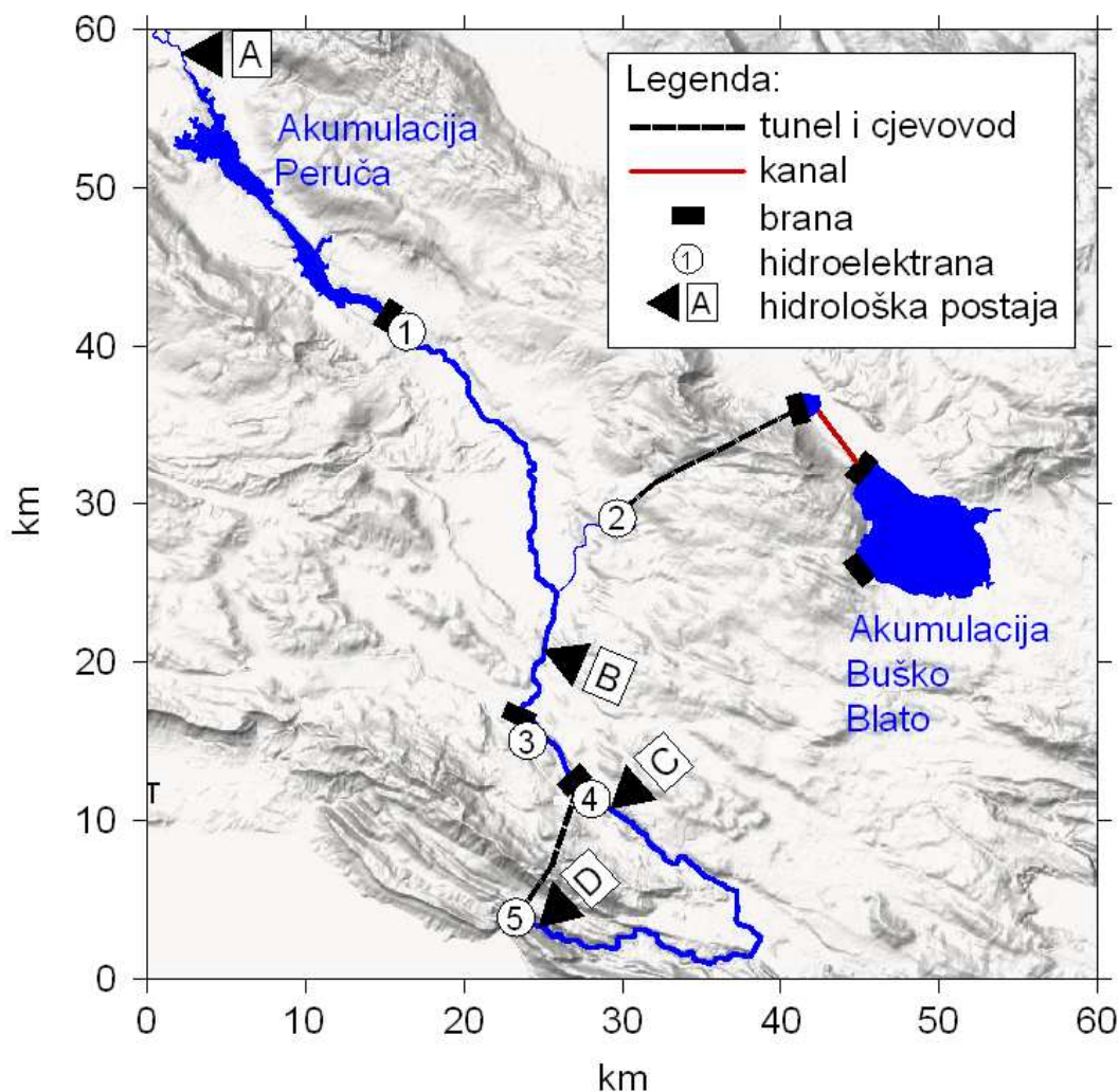
Slika 4.11 Površinski tok rijeke Cetine s hidrotehničkim objektima unutar sliva gdje su oznake (1) HE Peruča, (2) HE Orlovac, (3) HE Đale, (4) HE Kraljevac i (5) HE Zakučac. Značajne hidrološke postaje su označene sa (A) Vinalići, (B) Gardunska Mlinica, (C) Čikotina Lađa i (D) Tisne Stine.
