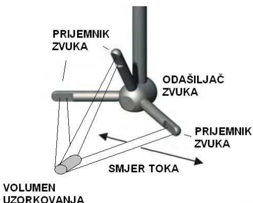
Slika 3.8 Akustična sonda ADV uređaja SONTEK Flowtracker
