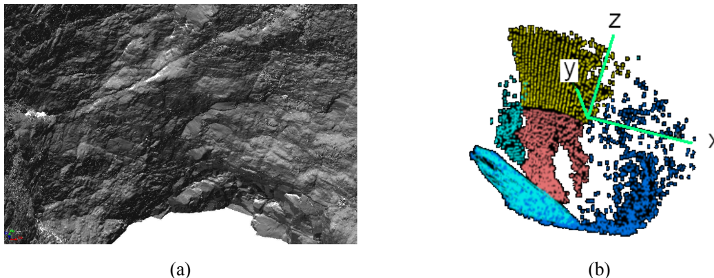
Slika 1.14 Oblak točkica mjereno TLS uređajem na a) primjeru Crvenog jezera te b) mjereno fotogrametrijskom metodom na primjeru Modrog jezera kod Imotskog
