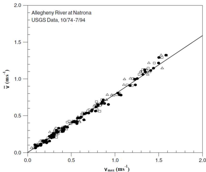
Slika 3.26 Prikazi odnosa v/v_{\max} za profil Natrona na rijeci Allegheny u SAD-i, \Phi(M)=0.81 (Chiu i Chen, 1999).
