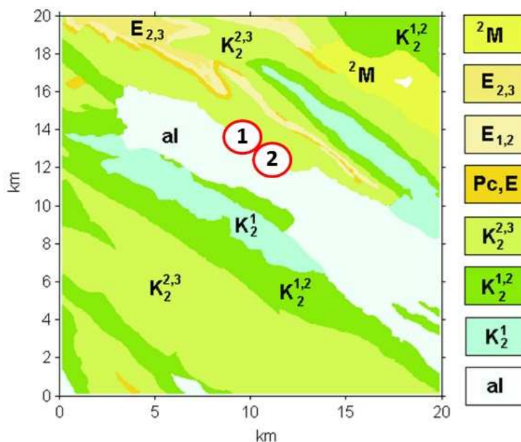
Slika 4.7 Litostratigrafska karta područja istraživanja oko Crvenog (1) i Modrog (2) jezera kod Imotskog. Tumač: (al) – aluvij, ( 2 M) – mastrihtski vapnenci, (E 2,3 ), (E 1,2 ), (Pc, E) – paleocenski i eocenski vapnenci, a (K 2 2,3 ), (K 2 1,2 ) – vapnenci gornje krede (OGK 1:100.000, list: Imotski).
