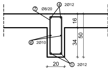
PRESJEK 1-1 M 1:25
