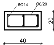
PRESJEK 3-3 M 1:25
