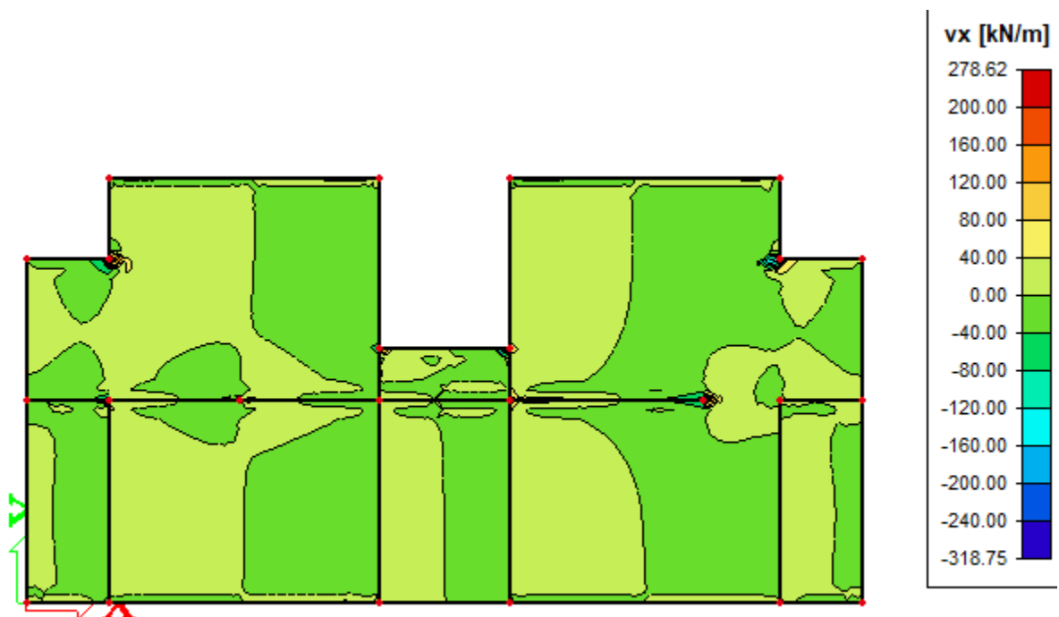
Slika 7.16 Poprečne sile V_{Ed,x} (kN/m) za GSN-1
