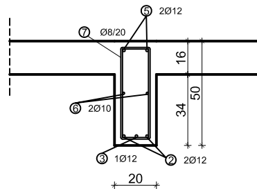
PRESJEK 3-3 M 1:25
