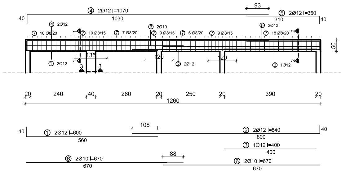
PRESJEK 1-1 M 1:25
