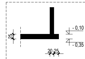
Presjek C-C
