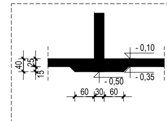
Presjek B-B
