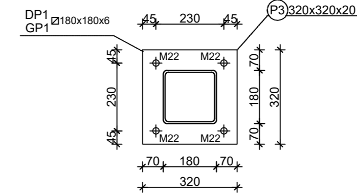
Presjek 4-4
