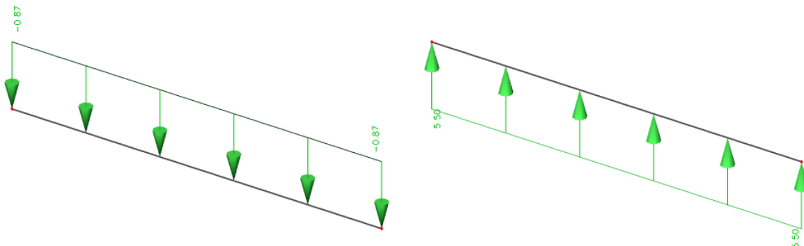
Slika 39 Djelovanje vjetra na krovne podrožnice
