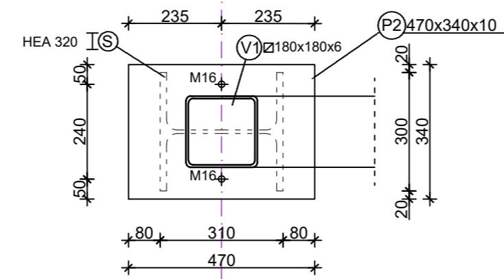
Presjek 2-2
