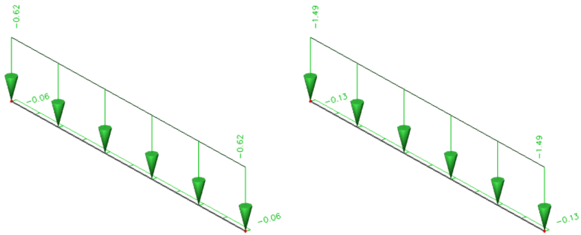
Slika 38 Djelovanja na krovnu podrožnicu
