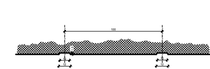
DETALJ KANELURA
