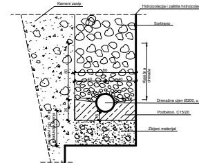
DETALJ DRENAŽE
