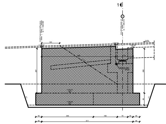
PRESJEK 6-6
