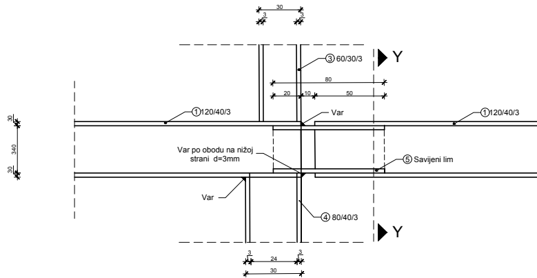
Detalj D 2 1:2
