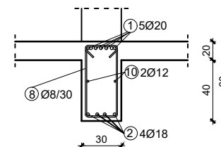
Presjek 3-3 (M 1:25)
