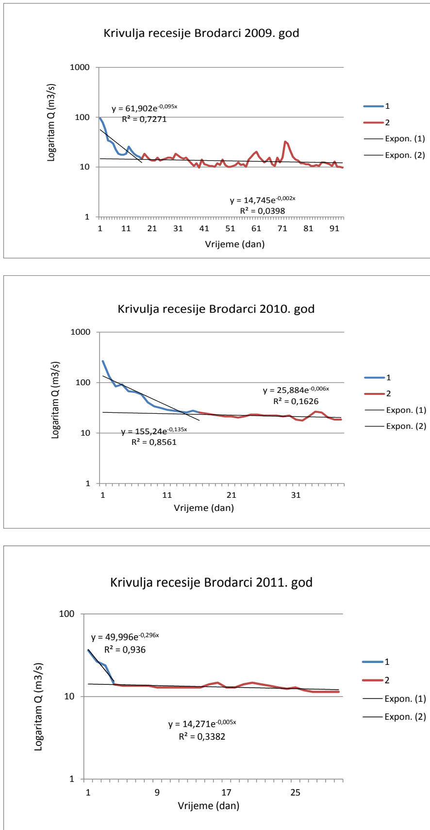
Slika 25. Krivulje recesije – rijeka Kupa (Brodarci)
